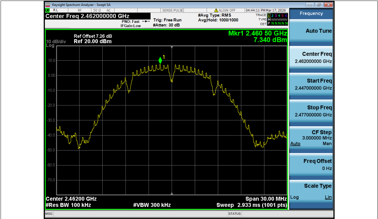
Band Edge NVNT b 2462MHz Ant1 Ref
