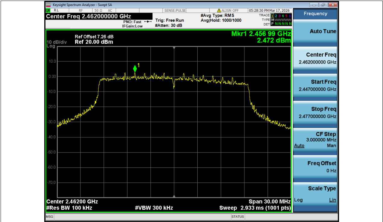
Band Edge NVNT ax20 2462MHz Ant1 Ref
