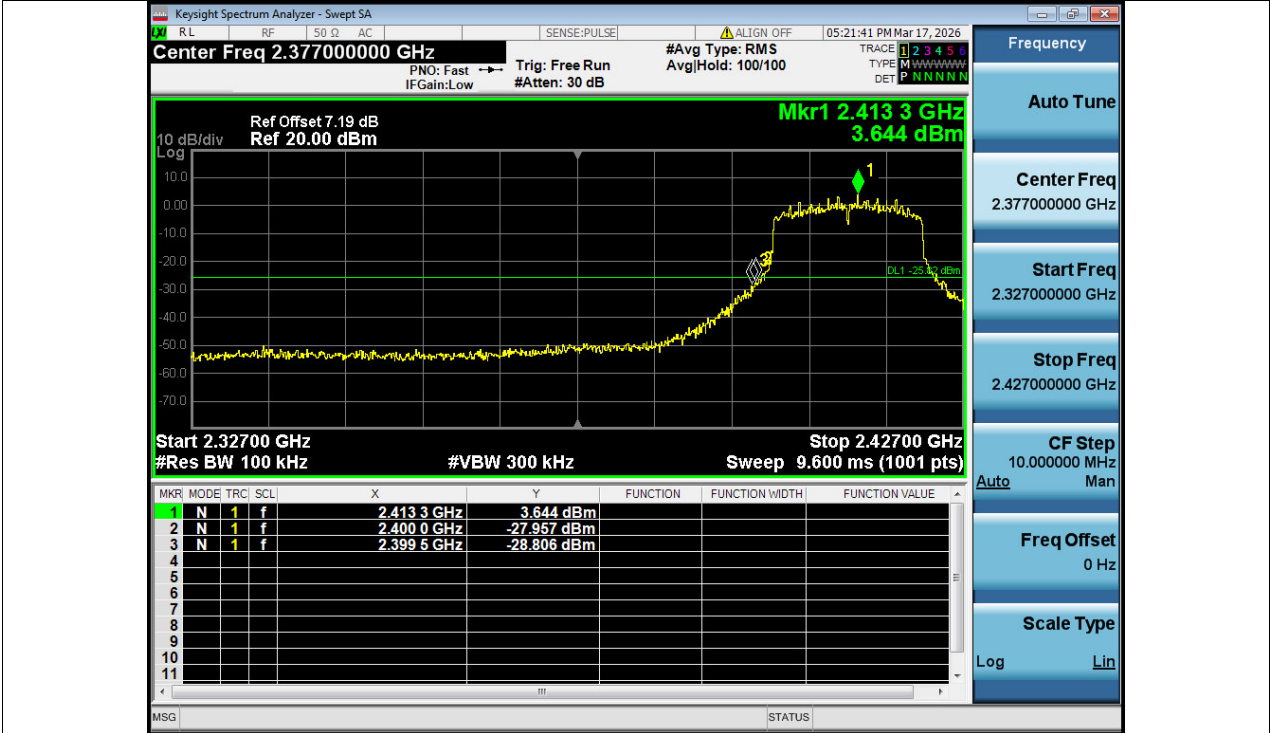
Band Edge NVNT ax20 2412MHz Ant1 Emission
