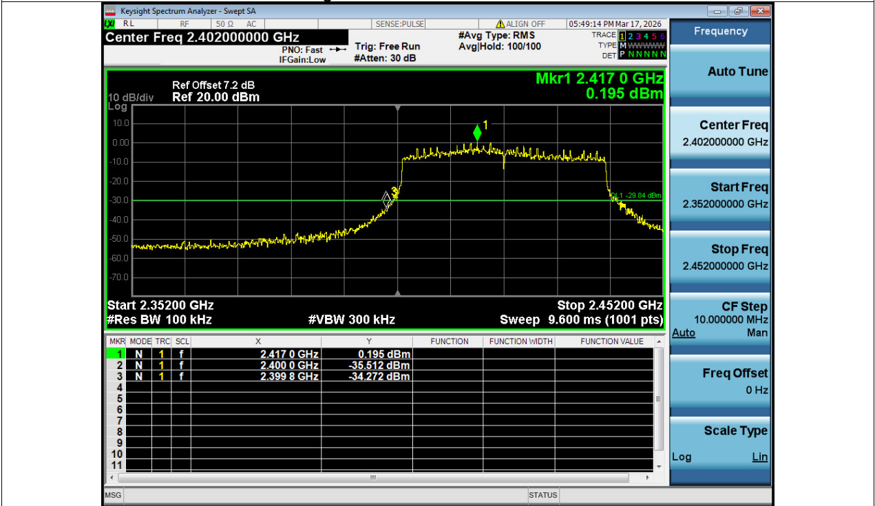
Band Edge NVNT ax40 2422MHz Ant1 Emission
