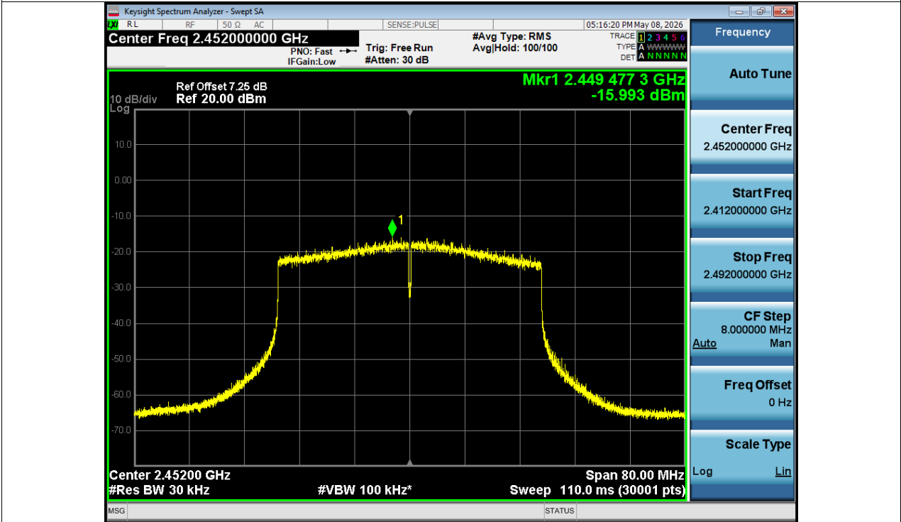
PSD NVNT ax40 2452MHz Ant1
