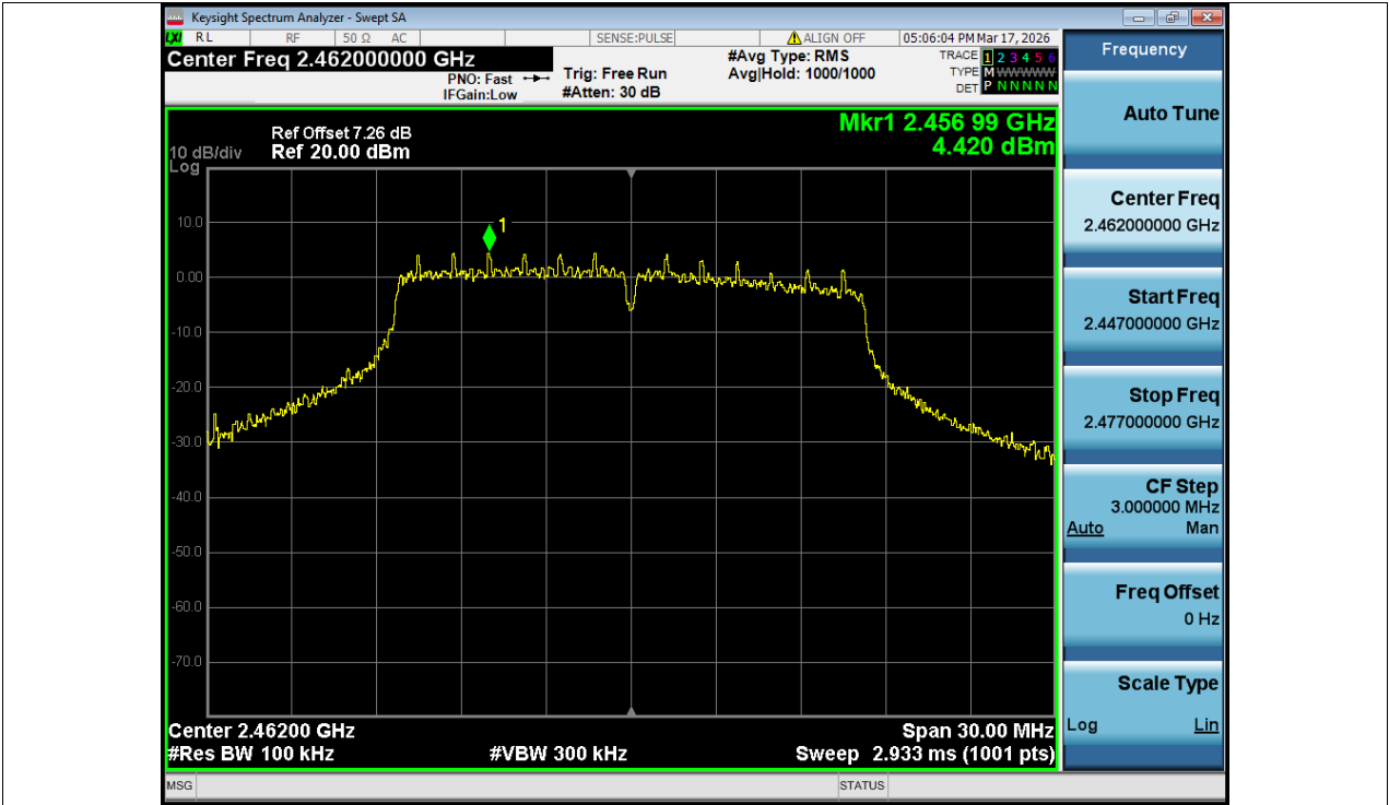
Band Edge NVNT g 2462MHz Ant1 Ref
