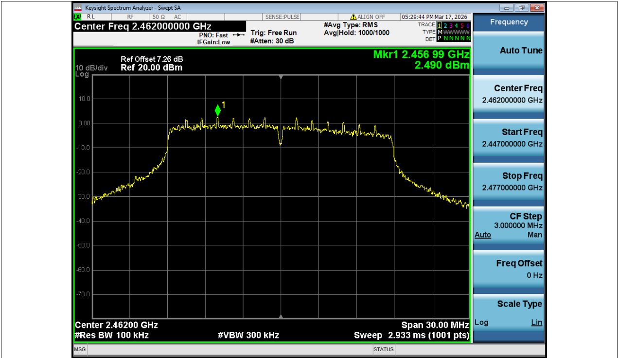
Band Edge NVNT n20 2462MHz Ant1 Ref
