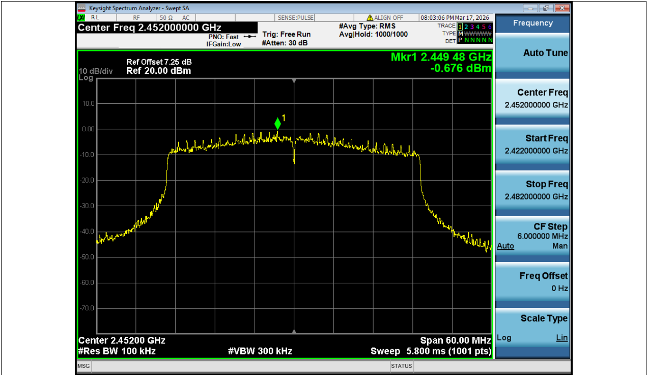
Band Edge NVNT ax40 2452MHz Ant1 Ref
