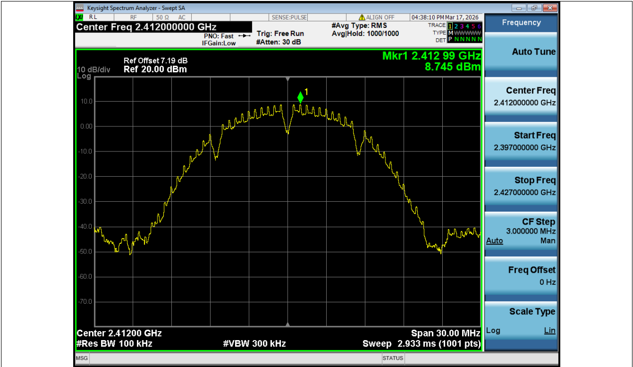
Band Edge NVNT b 2412MHz Ant1 Ref
