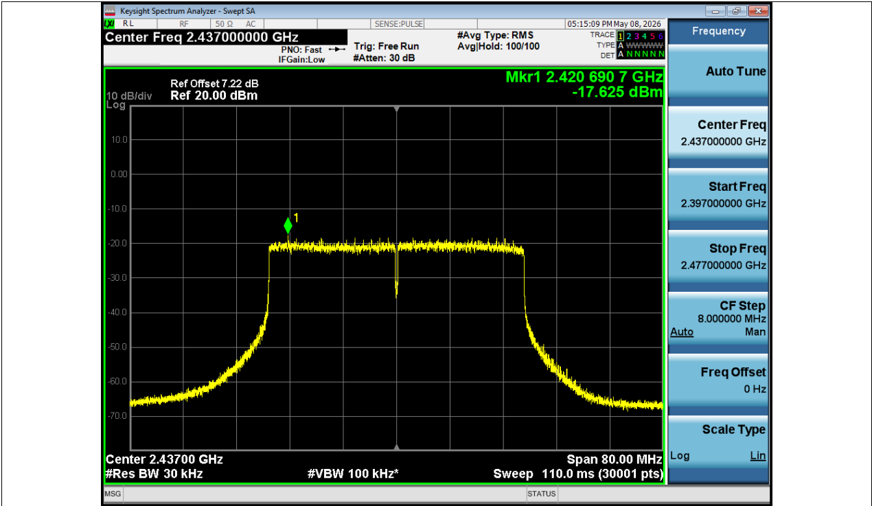
PSD NVNT ax40 2437MHz Ant1
