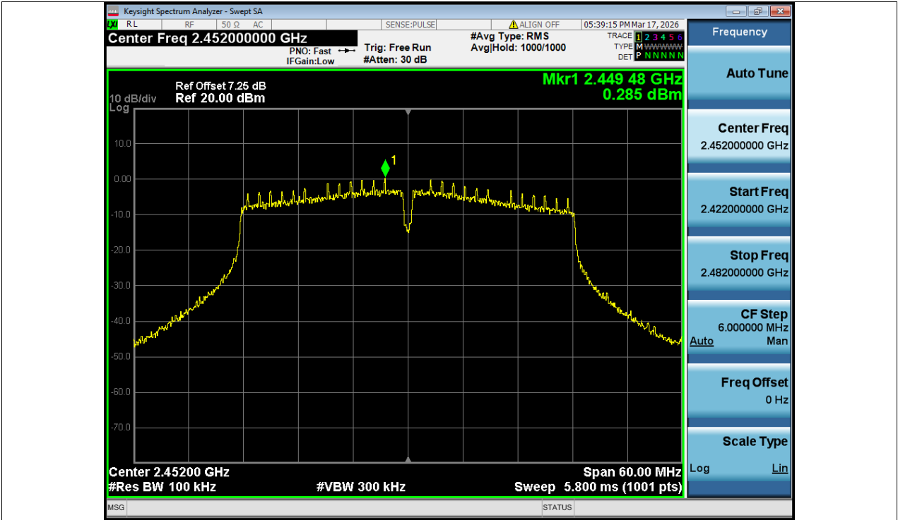
Band Edge NVNT n40 2452MHz Ant1 Ref
