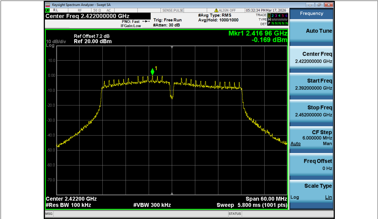
Band Edge NVNT n40 2422MHz Ant1 Ref
