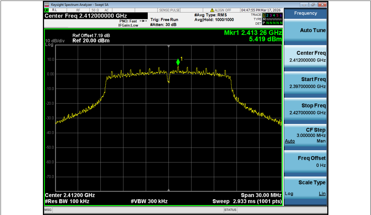
Band Edge NVNT g 2412MHz Ant1 Ref
