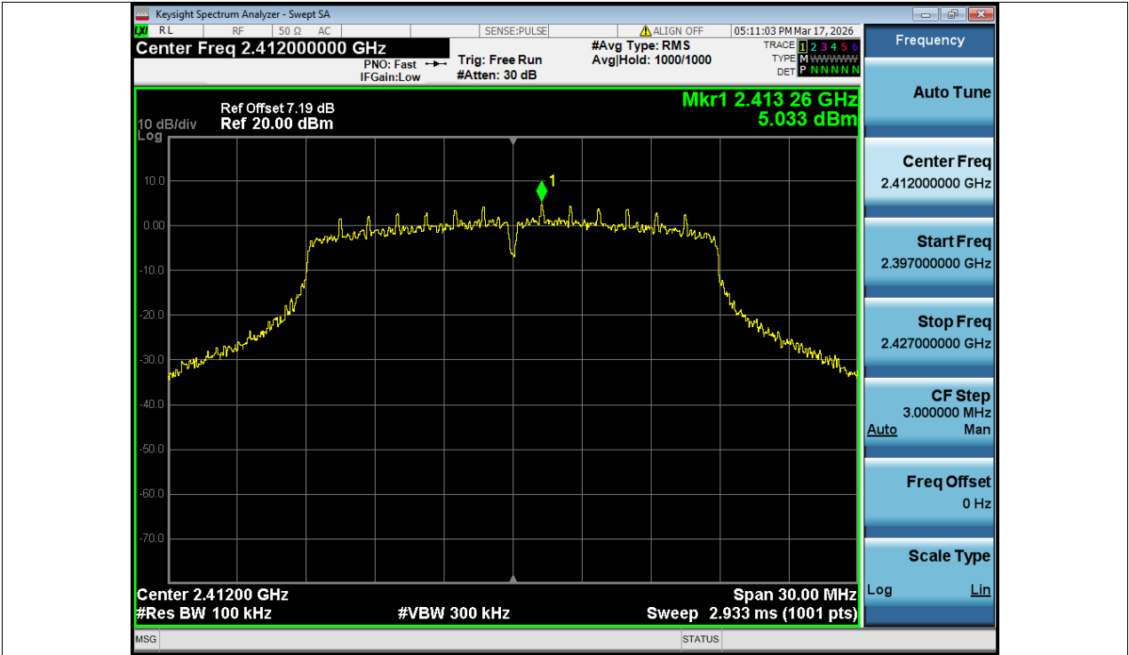
Band Edge NVNT n20 2412MHz Ant1 Ref
