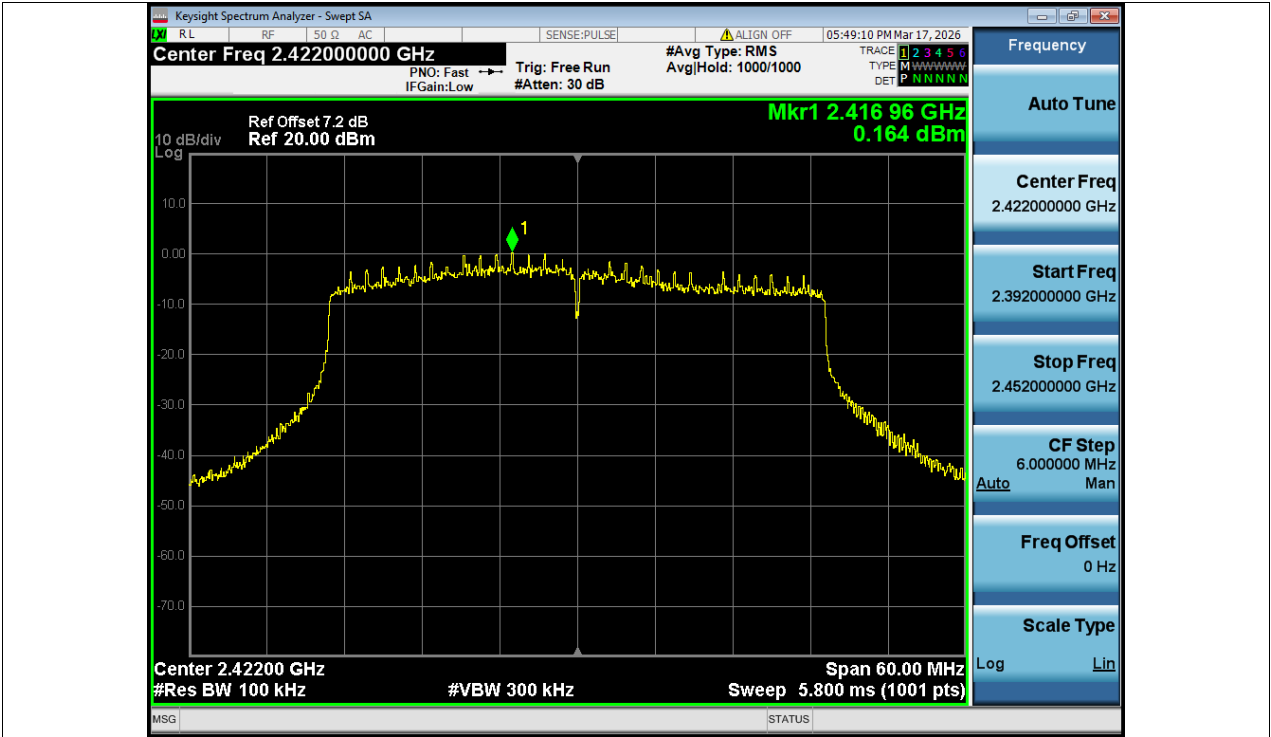
Band Edge NVNT ax40 2422MHz Ant1 Ref
