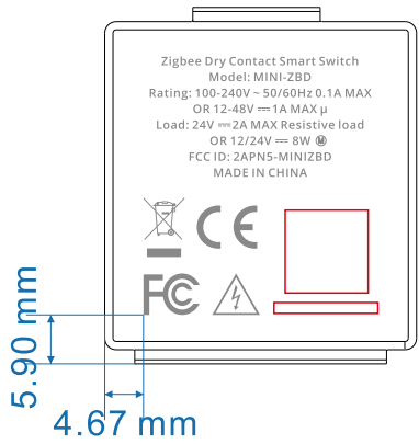
镭雕位置
