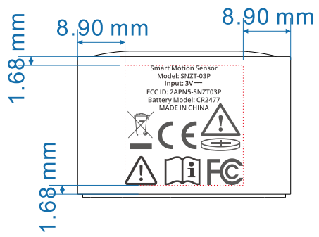
按钮孔背面
