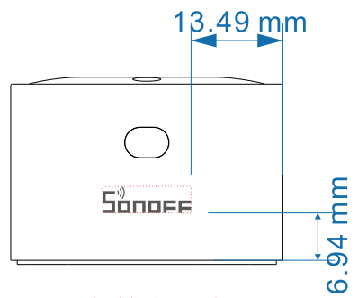
按钮孔正面
