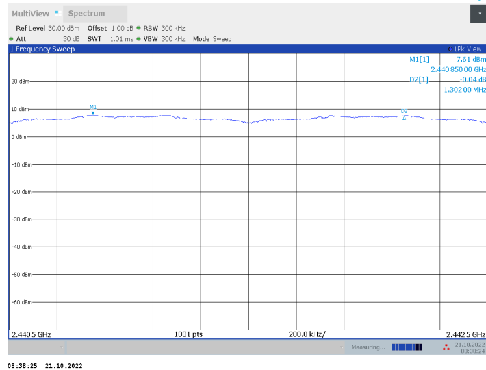
2DH5_Ant2_Hop
