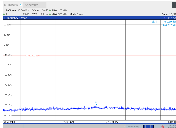
DH5_Ant2_2402_30~1000
