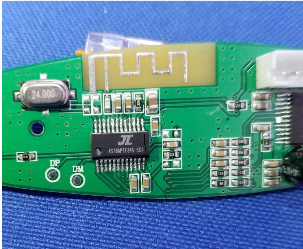
(8) EUT Photo
