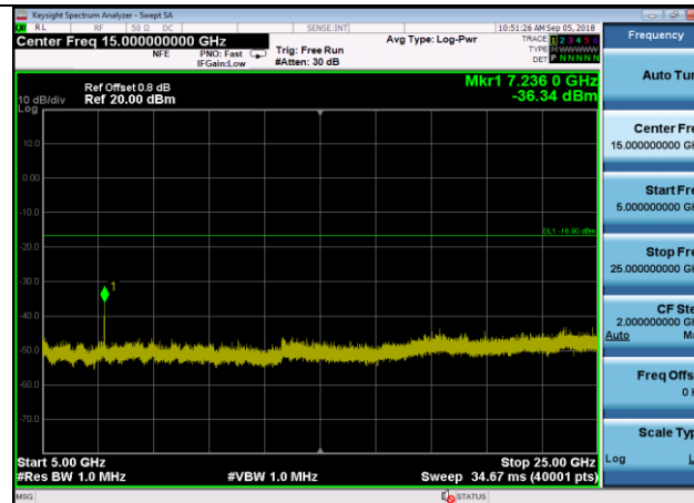
802.11b,2412MHz,Ant0,Plot 5,5000MHz~25000MHz
