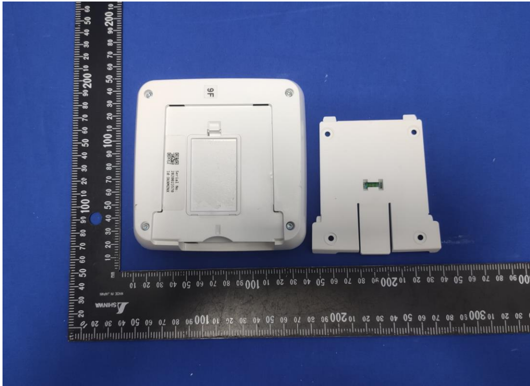
(2) EUT Photo
