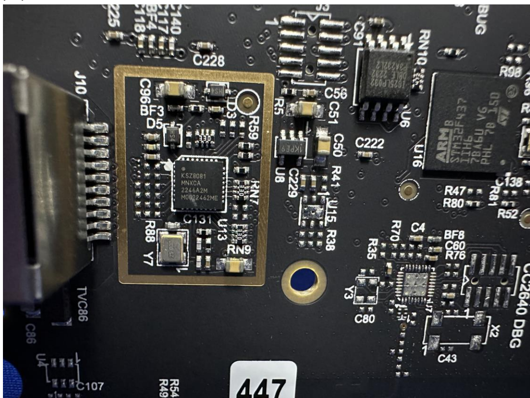
(12) EUT Photo
