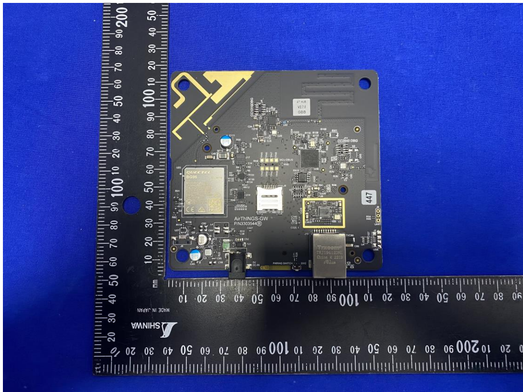
(6) EUT Photo
