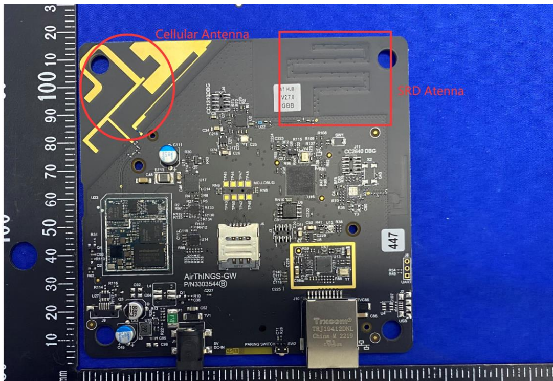
(8) EUT Photo
