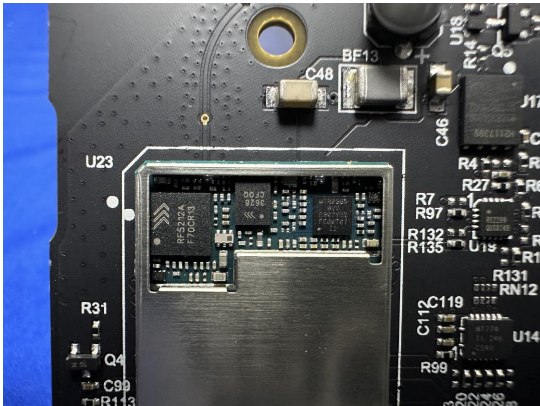
(14) EUT Photo
