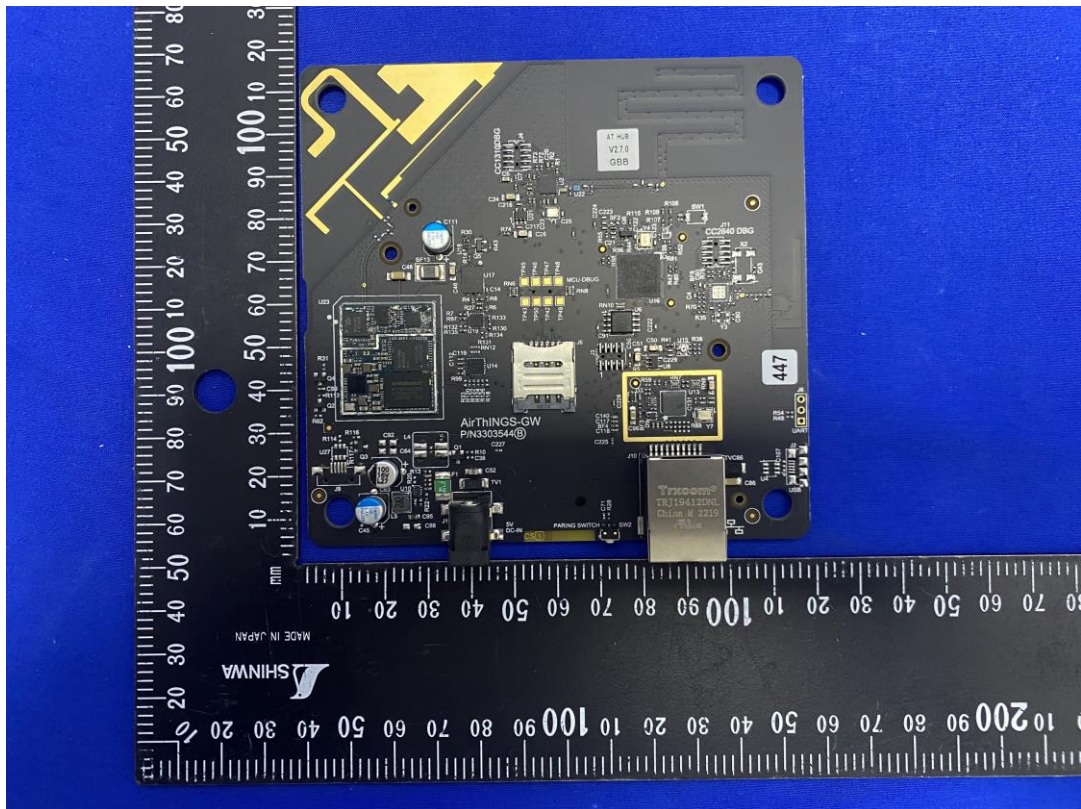
(8) EUT Photo
