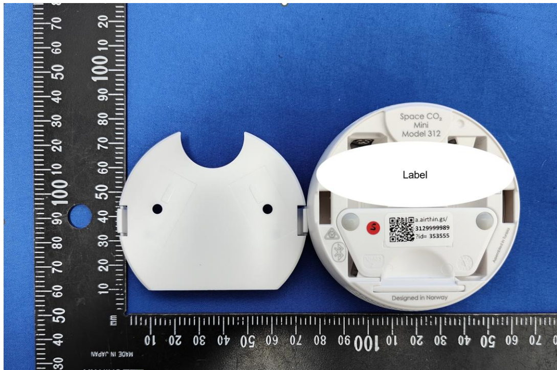
(7)EUT Photo
