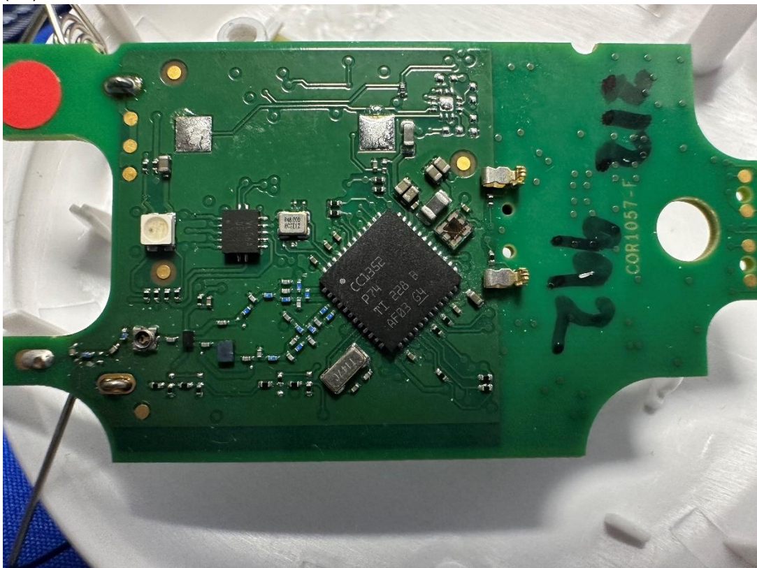
(10) EUT Photo
