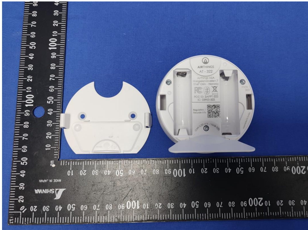
(8)EUT Photo
