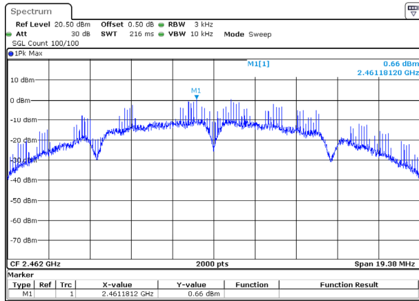
802.11b_2462MHz
