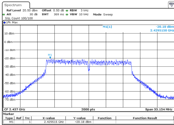
802.11g_2437MHz
