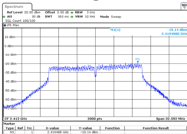
802.11n20_2412MHz
