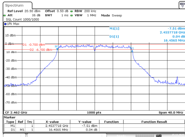
802.11n20_2462MHz
