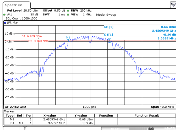
802.11b_2462MHz
