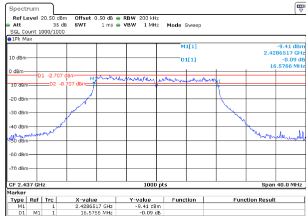
802.11n20_2437MHz
