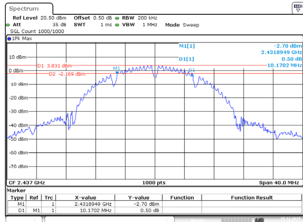
802.11b_2437MHz
