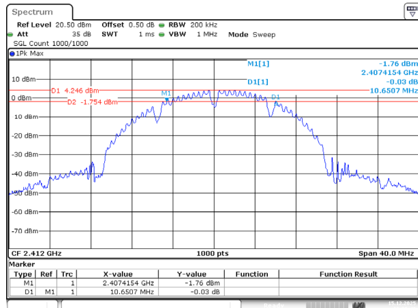
802.11b_2412MHz
