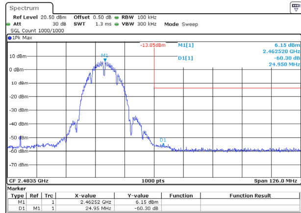
802.11b_2462MHz
