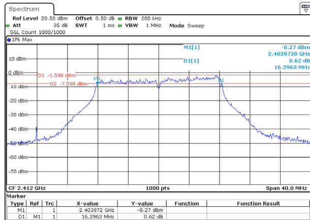
802.11n20_2412MHz
