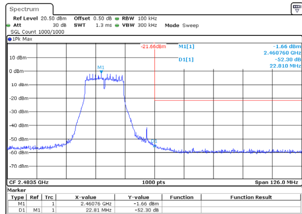
802.11n20_2462MHz
