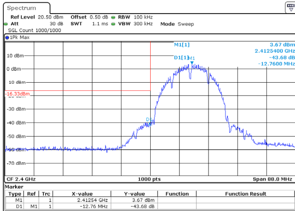
802.11b_2412MHz
