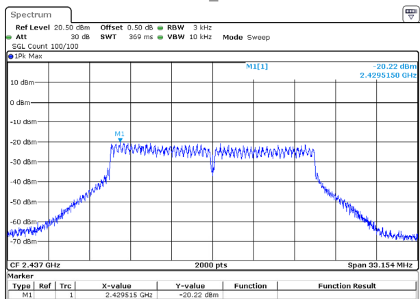
802.11n20_2437MHz
