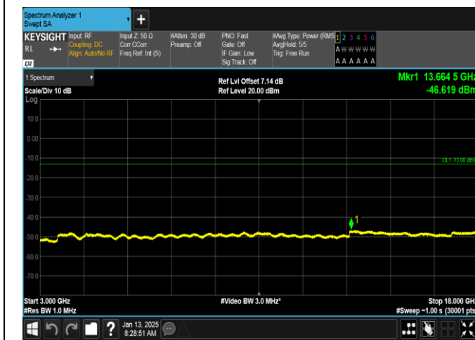
GSM1900-810-0-3000~18000MHz-PASS
