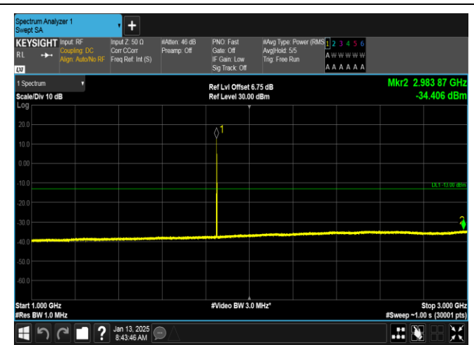
GPRS1900-512-0-1000~3000MHz-PASS
