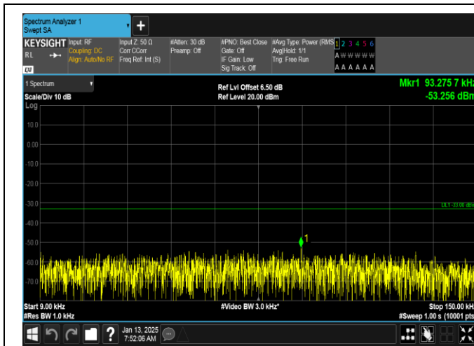
GSM850-251-5-0.009~0.15MHz-PASS
