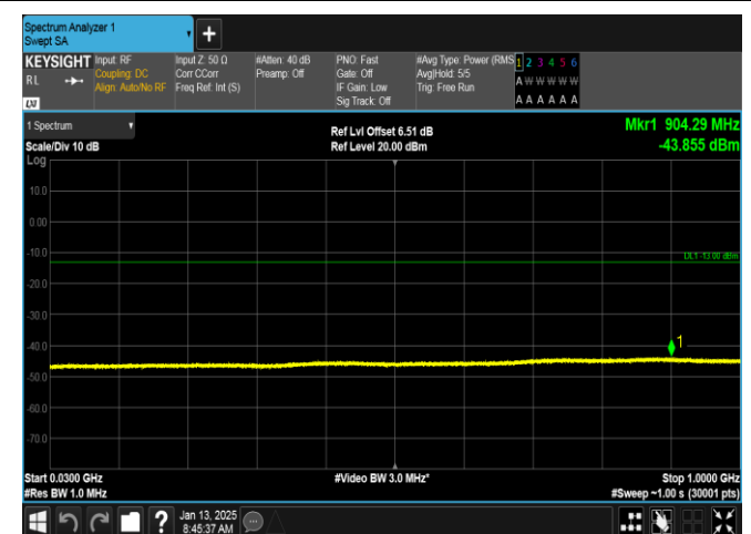
GPRS1900-810-0-30~1000MHz-PASS
