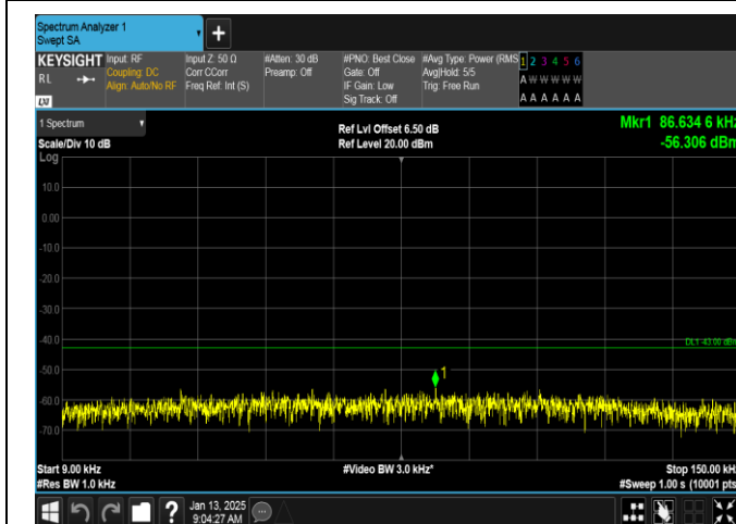
EGPRS1900-810-2-0.009~0.15MHz-PASS
