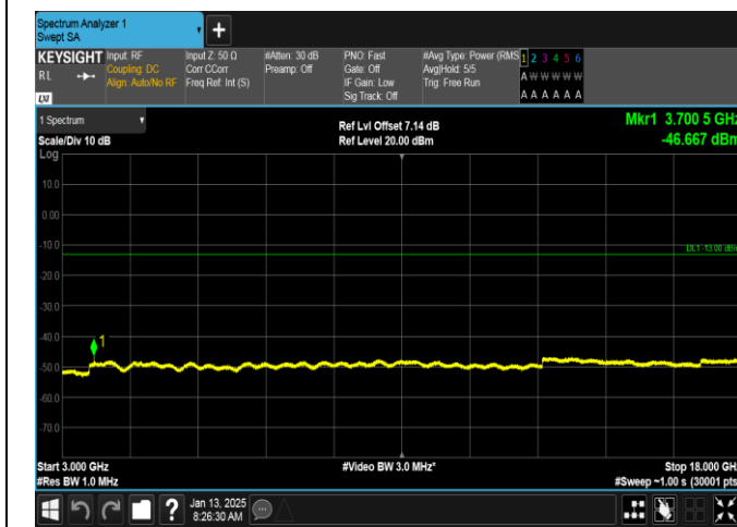
GSM1900-512-0-3000~18000MHz-PASS
