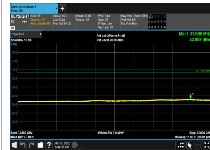
GPRS1900-661-0-30~1000MHz-PASS
