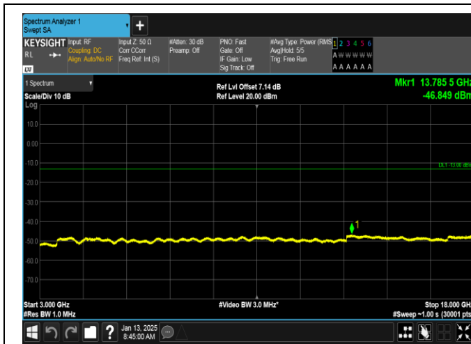
GPRS1900-661-0-3000~18000MHz-PASS
