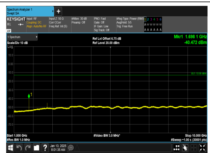
GPRS850-251-5-1000~10000MHz-PASS
