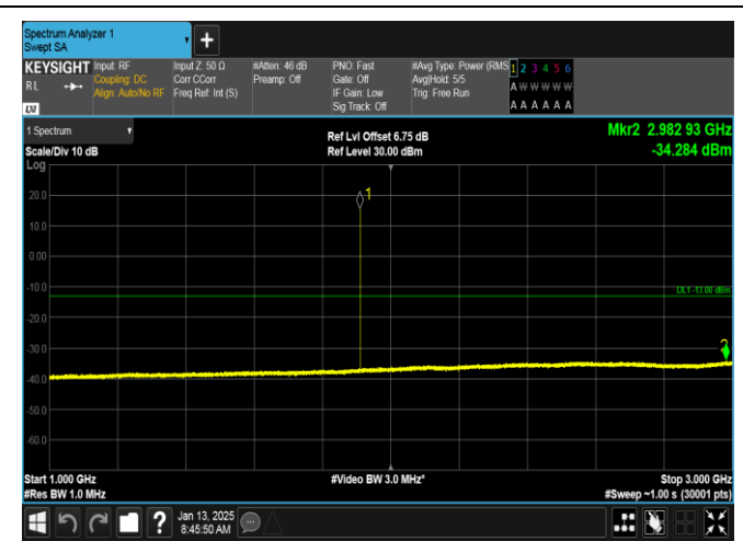
GPRS1900-810-0-1000~3000MHz-PASS
