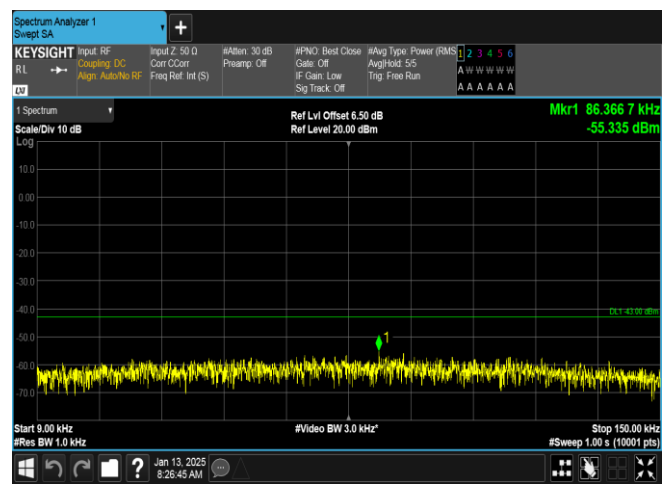
GSM1900-661-0-0.009~0.15MHz-PASS
