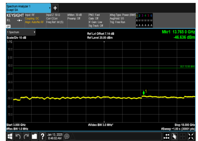
GPRS1900-810-0-3000~18000MHz-PASS
