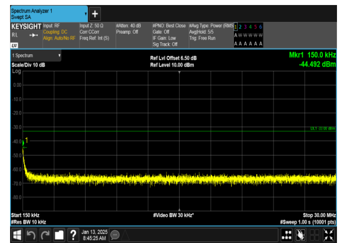
GPRS1900-810-0-0.15~30MHz-PASS
