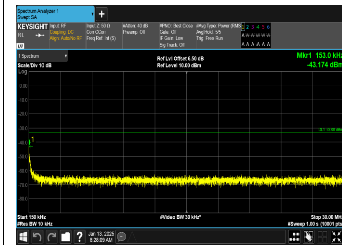
GSM1900-810-0-0.15~30MHz-PASS
