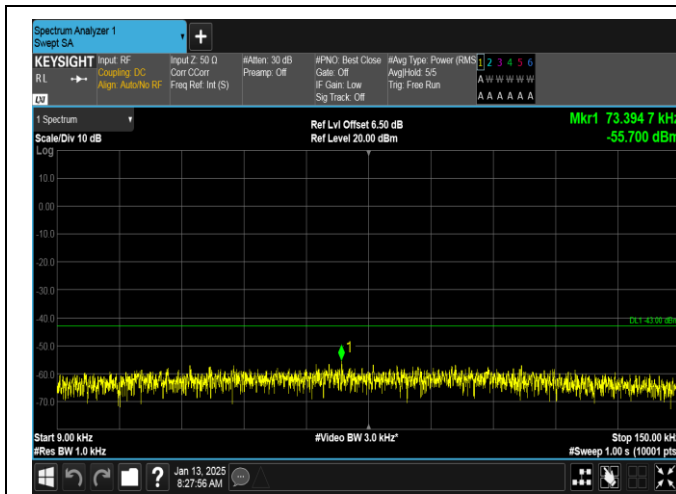
GSM1900-810-0-0.009~0.15MHz-PASS
