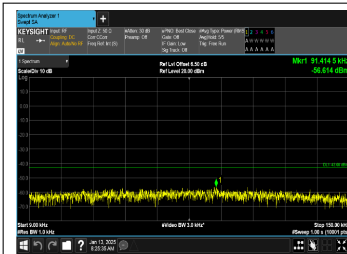
GSM1900-512-0-0.009~0.15MHz-PASS
