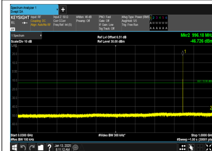
EGPRS850-251-8-30~1000MHz-PASS
