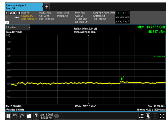
GPRS1900-512-0-3000~18000MHz-PASS
