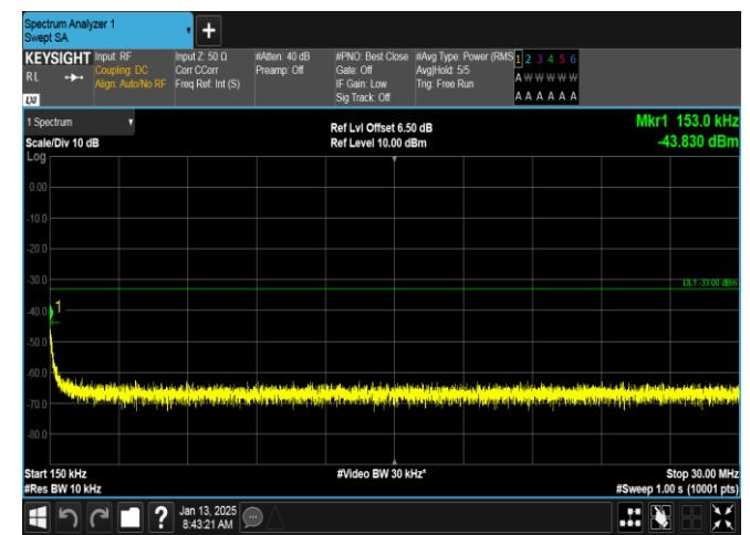
GPRS1900-512-0-0.15~30MHz-PASS
