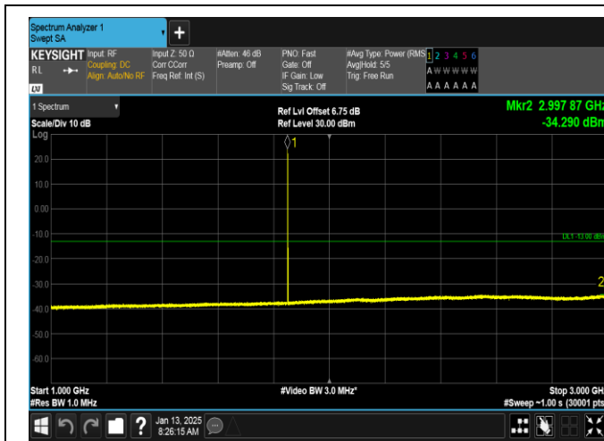
GSM1900-512-0-1000~3000MHz-PASS
