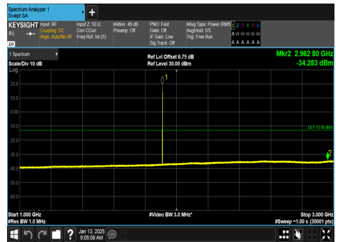
EGPRS1900-810-2-1000~3000MHz-PASS
