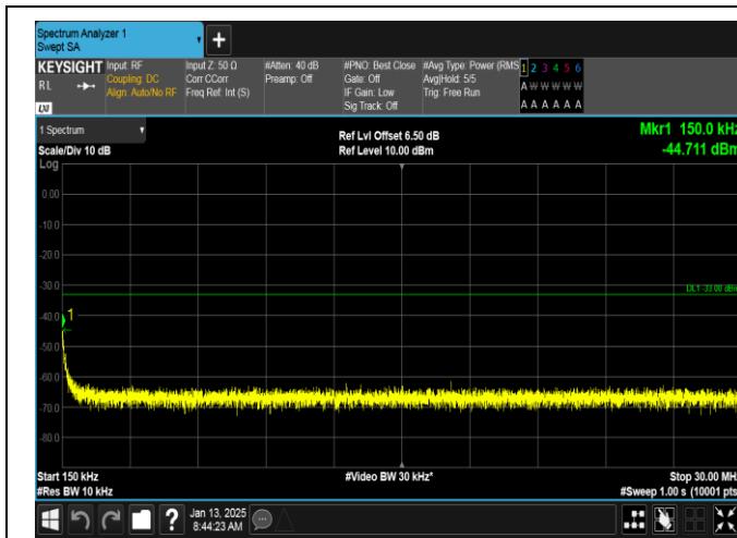
GPRS1900-661-0-0.15~30MHz-PASS
