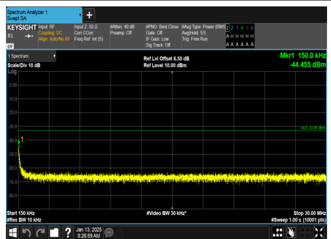
GSM1900-661-0-0.15~30MHz-PASS
