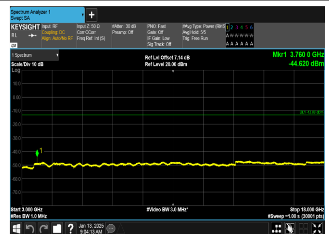
EGPRS1900-661-2-3000~18000MHz-PASS
