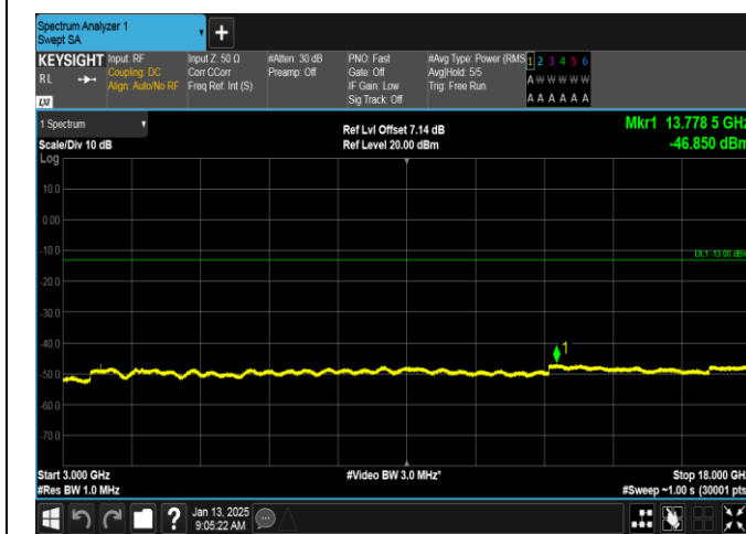
EGPRS1900-810-2-3000~18000MHz-PASS
