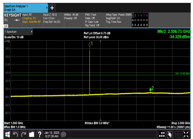
GSM1900-661-0-1000~3000MHz-PASS
