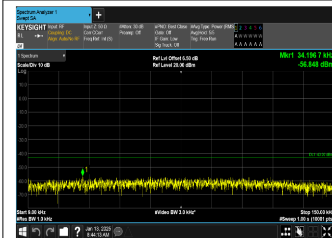
GPRS1900-661-0-0.009~0.15MHz-PASS
