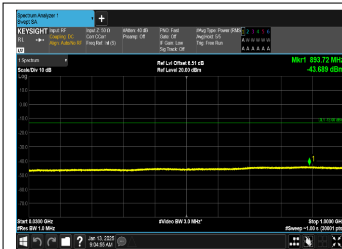
EGPRS1900-810-2-30~1000MHz-PASS
