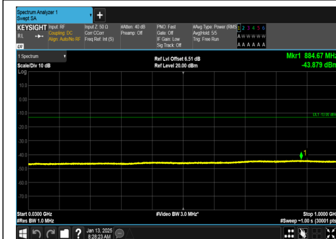
GSM1900-810-0-30~1000MHz-PASS
