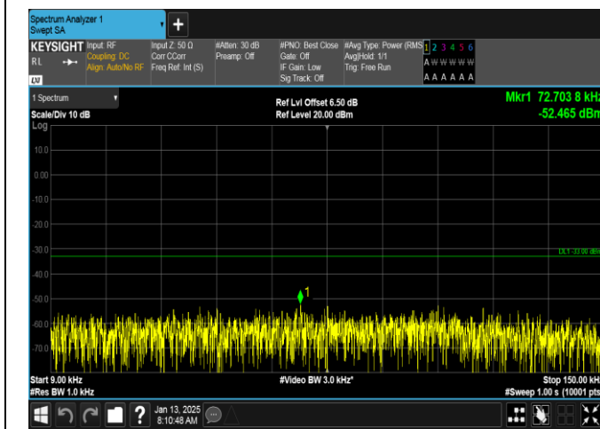
EGPRS850-251-8-0.009~0.15MHz-PASS
