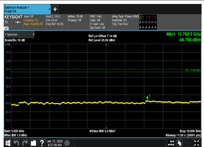
GSM1900-661-0-3000~18000MHz-PASS
