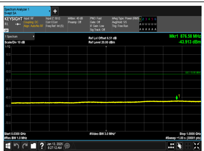
GSM1900-661-0-30~1000MHz-PASS
