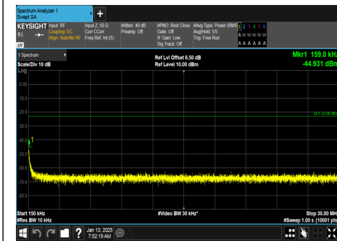
GSM850-251-5-0.15~30MHz-PASS
