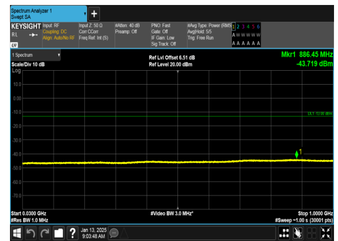
EGPRS1900-661-2-30~1000MHz-PASS
