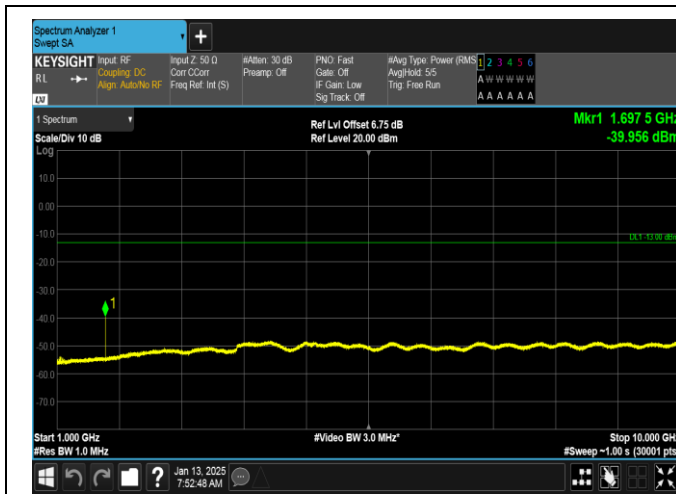
GSM850-251-5-1000~10000MHz-PASS
