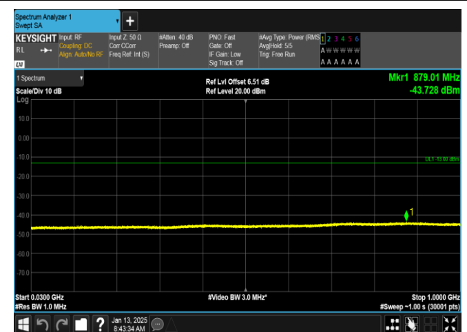
GPRS1900-512-0-30~1000MHz-PASS
