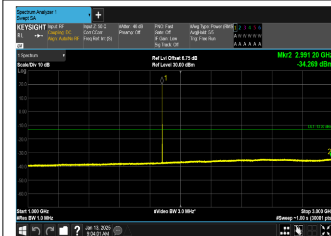
EGPRS1900-661-2-1000~3000MHz-PASS
