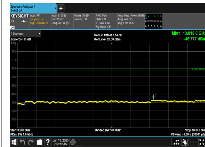
EGPRS1900-512-2-3000~18000MHz-PASS
