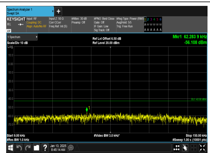
GPRS1900-810-0-0.009~0.15MHz-PASS
