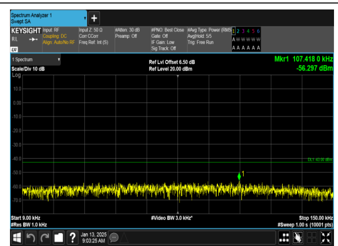
EGPRS1900-661-2-0.009~0.15MHz-PASS
