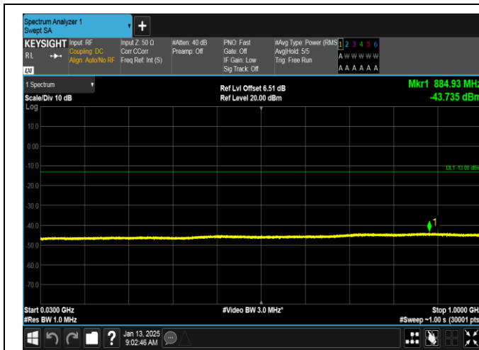
EGPRS1900-512-2-30~1000MHz-PASS
