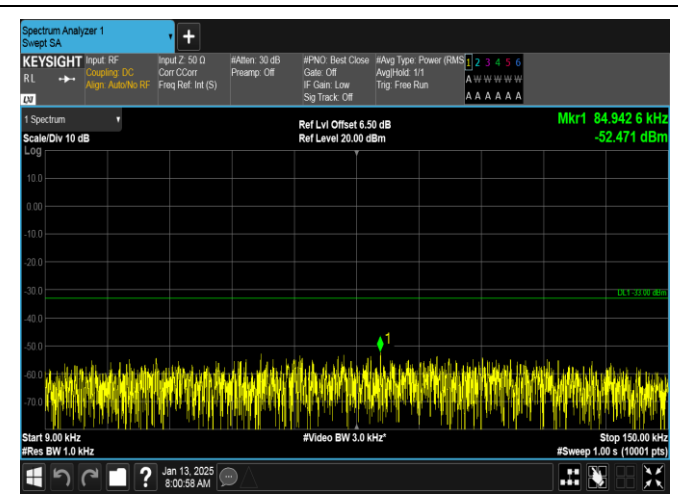
GPRS850-251-5-0.009~0.15MHz-PASS
