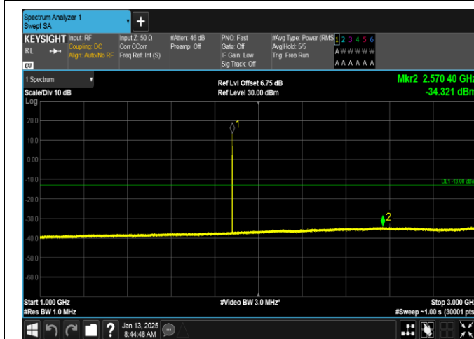
GPRS1900-661-0-1000~3000MHz-PASS
