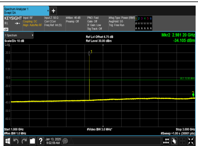
EGPRS1900-512-2-1000~3000MHz-PASS
