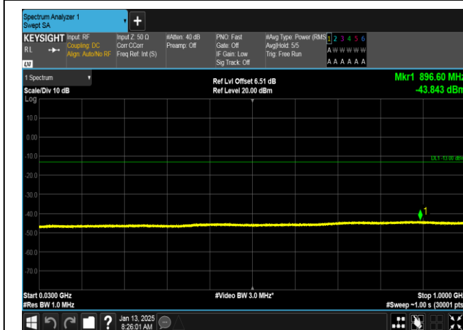
GSM1900-512-0-30~1000MHz-PASS
