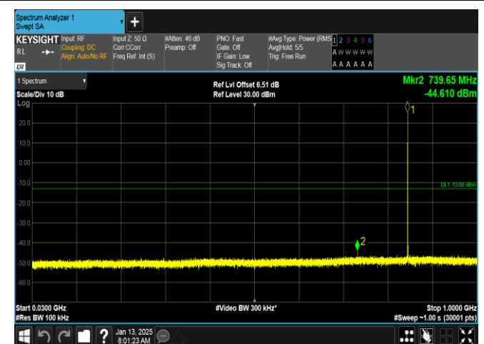
GPRS850-251-5-30~1000MHz-PASS
