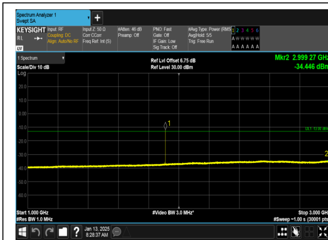
GSM1900-810-0-1000~3000MHz-PASS
