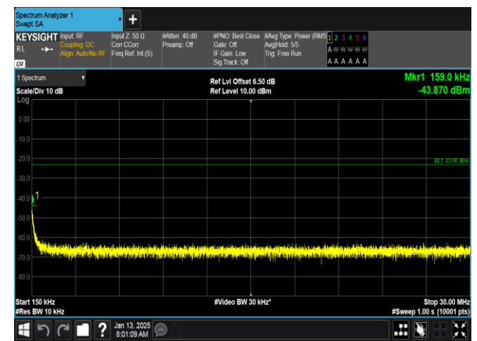
GPRS850-251-5-0.15~30MHz-PASS
