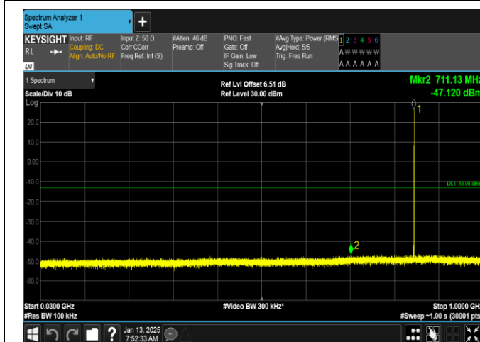
GSM850-251-5-30~1000MHz-PASS
