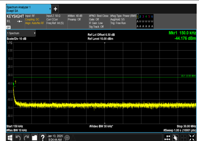
EGPRS1900-810-2-0.15~30MHz-PASS
