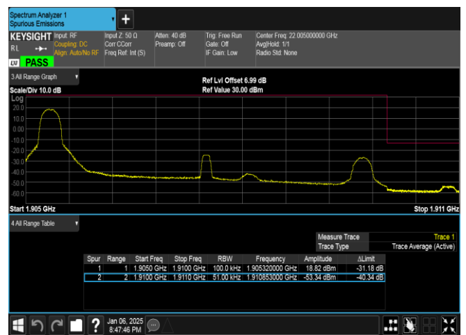
Band2-5MHz-QPSK-19175-1RB#0-PASS
