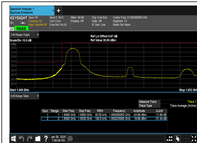
Band2-3MHz-QPSK-18615-1RB#0-PASS
