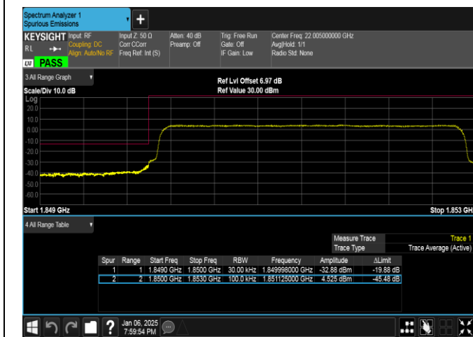
Band2-3MHz-QPSK-18615-15RB#0-PASS
