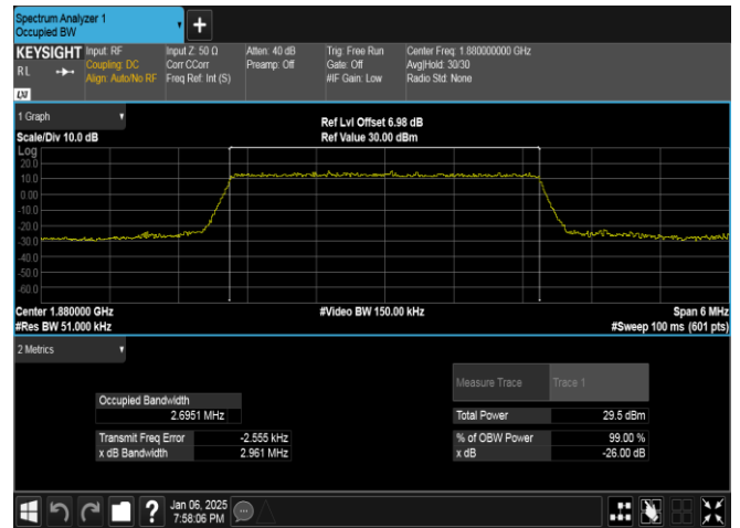
Band2-3MHz-QPSK-18900-15RB#0-PASS
