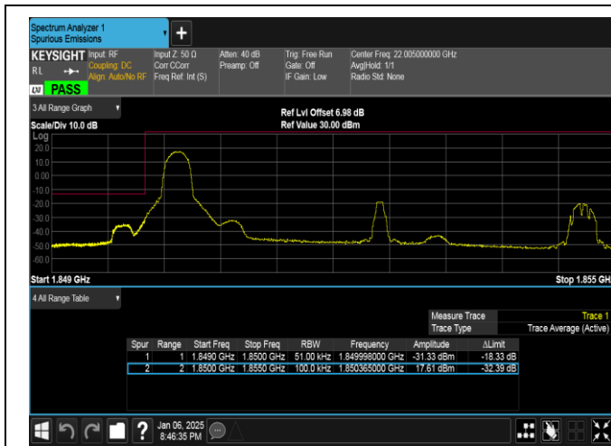
Band2-5MHz-16QAM-18625-1RB#0-PASS
