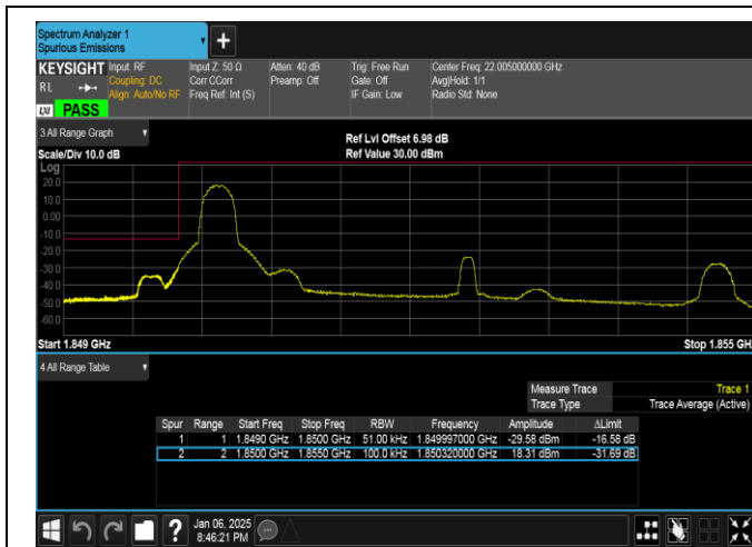
Band2-5MHz-QPSK-18625-1RB#0-PASS
