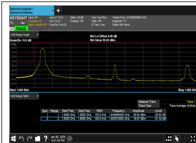
Band2-10MHz-QPSK-18650-1RB#0-PASS
