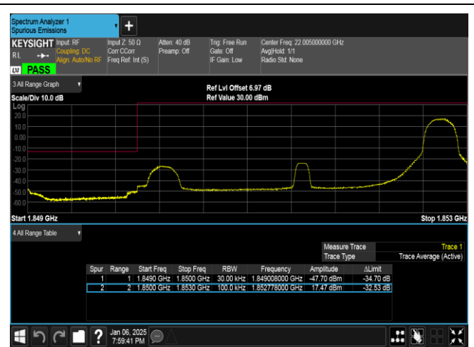
Band2-3MHz-16QAM-18615-1RB#14-PASS
