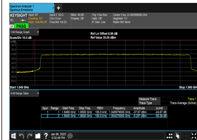
Band2-10MHz-QPSK-18650-50RB#0-PASS
