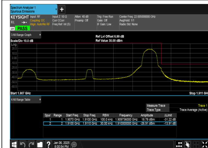
Band2-3MHz-QPSK-19185-1RB#14-PASS
