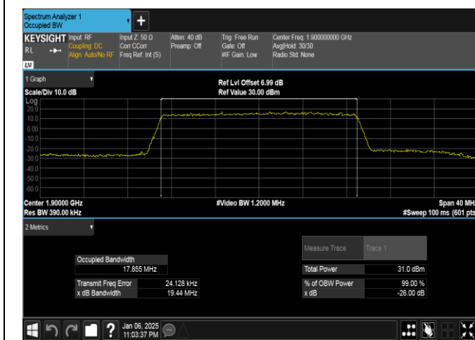
Band2-20MHz-QPSK-19100-100RB#0-PASS
