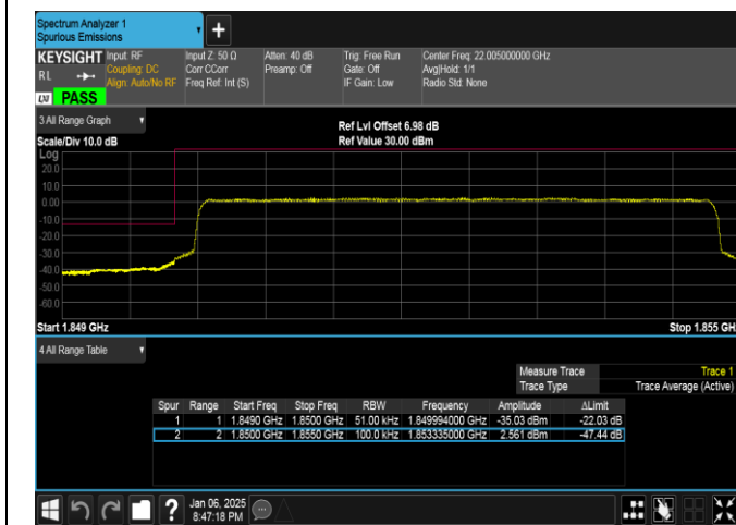
Band2-5MHz-QPSK-18625-25RB#0-PASS
