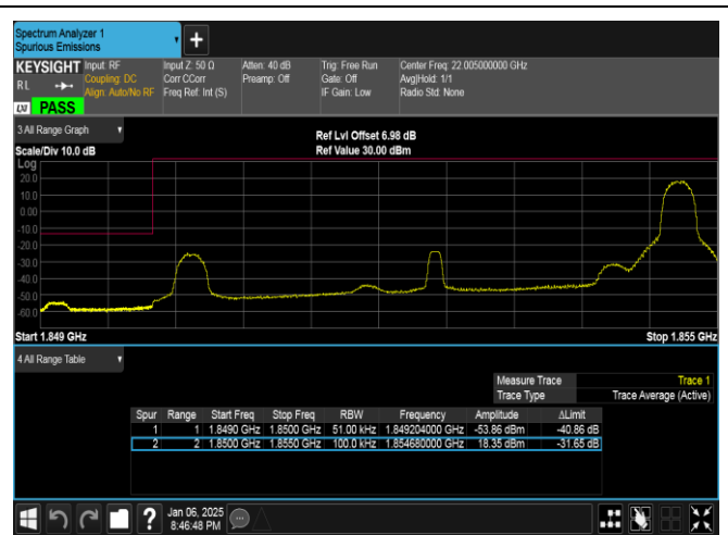
Band2-5MHz-QPSK-18625-1RB#24-PASS
