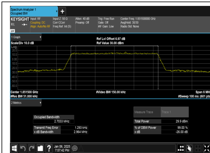
Band2-3MHz-QPSK-18615-15RB#0-PASS
