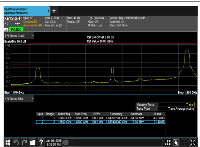
Band2-10MHz-QPSK-18650-1RB#49-PASS
