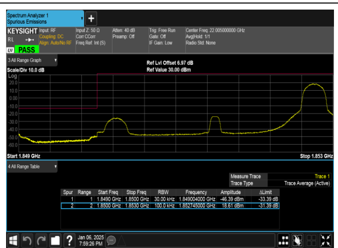
Band2-3MHz-QPSK-18615-1RB#14-PASS
