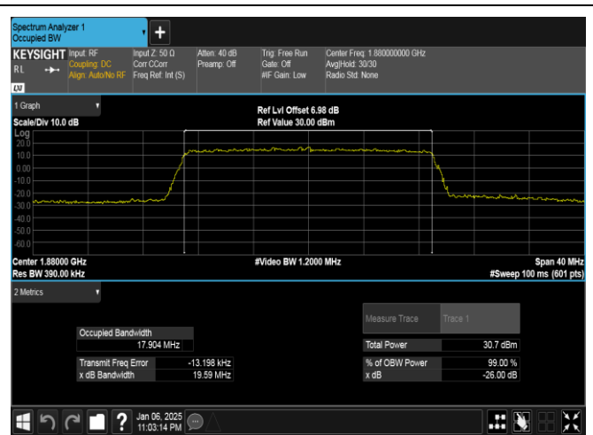
Band2-20MHz-QPSK-18900-100RB#0-PASS
