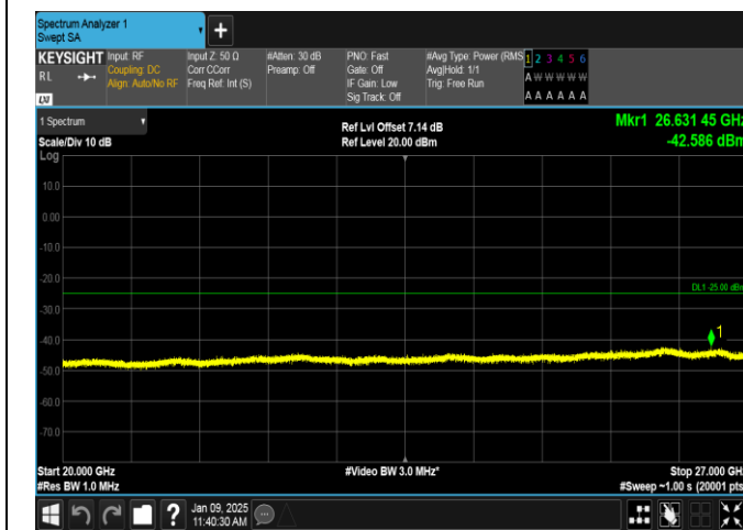
Band38-15MHz-QPSK-38175-1RB#0-20000~27000-PASS
