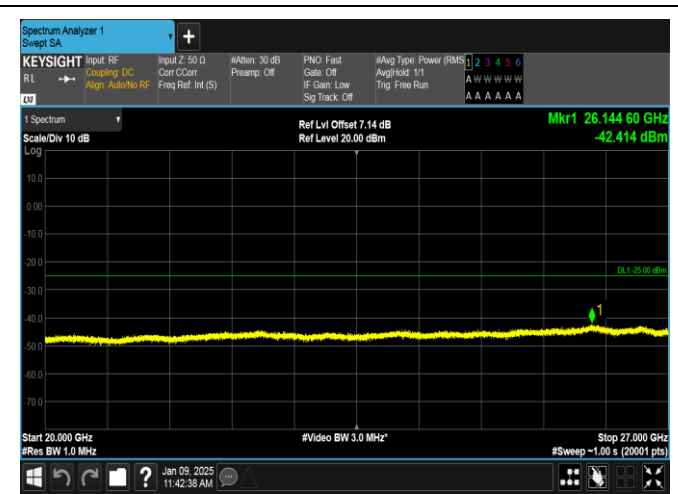
Band38-15MHz-QPSK-38175-1RB#74-20000~27000-PASS
