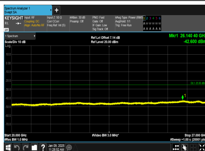
Band38-15MHz-16QAM-37825-1RB#0-20000~27000-PASS
