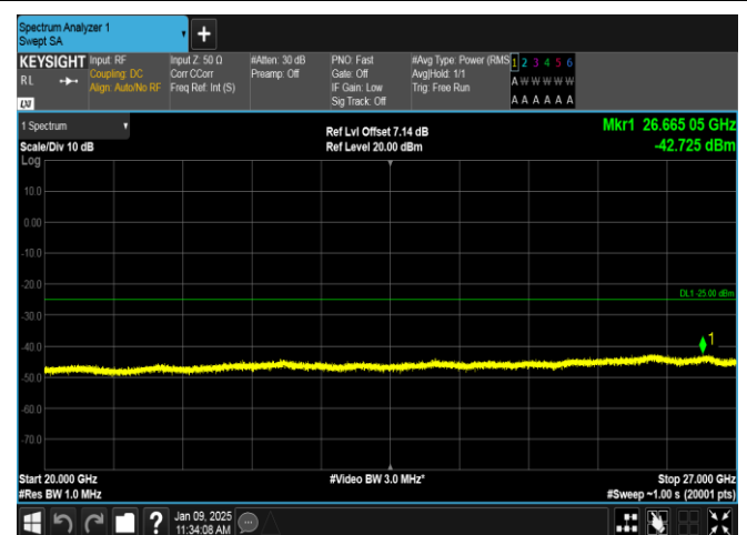
Band38-15MHz-QPSK-38000-1RB#0-20000~27000-PASS
