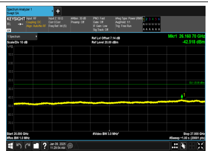
Band38-15MHz-QPSK-37825-1RB#74-20000~27000-PASS
