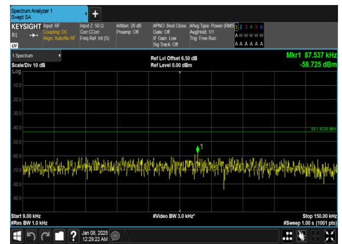
Band4-20MHz-QPSK-20175-1RB#0-0.009~0.15-PASS
