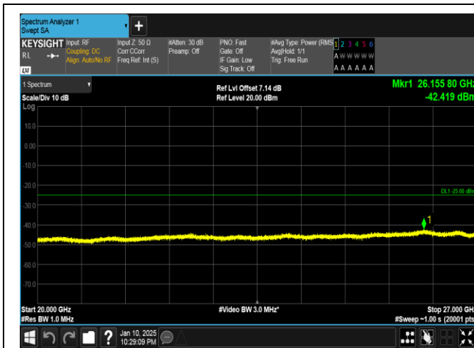
Band41-20MHz-QPSK-41490-100RB#0-20000~27000-PASS
