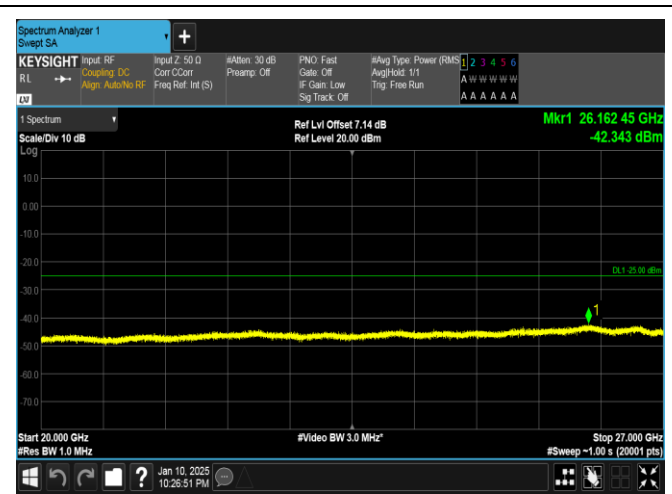
Band41-20MHz-QPSK-41490-1RB#99-20000~27000-PASS
