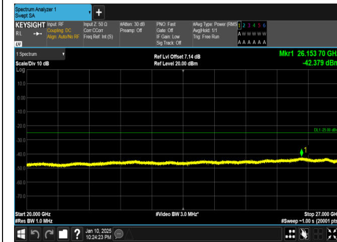
Band41-20MHz-QPSK-41490-1RB#0-20000~27000-PASS
