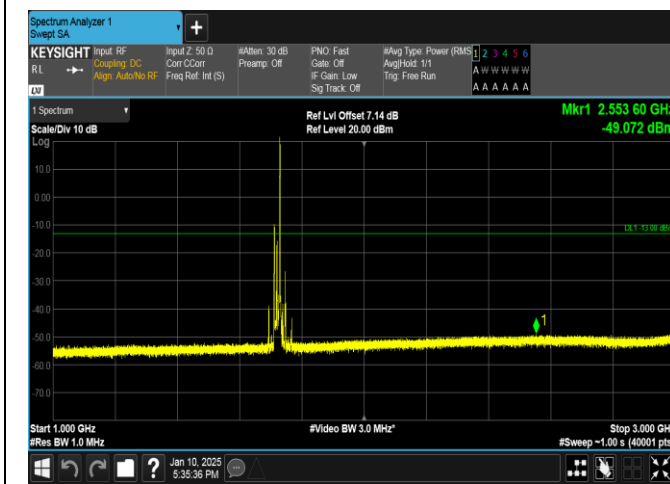
Band66-20MHz-QPSK-132072-1RB#99-1000~3000-PASS
