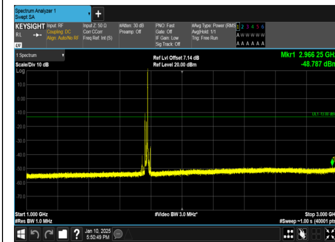
Band66-20MHz-QPSK-132572-1RB#99-1000~3000-PASS
