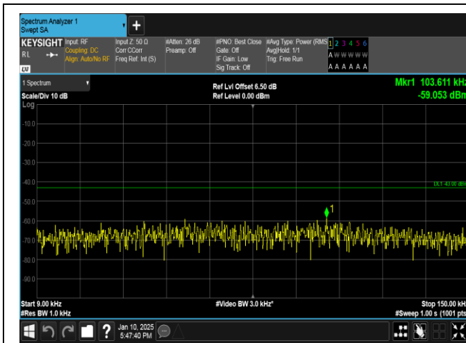
Band66-20MHz-QPSK-132572-1RB#0-0.009~0.15-PASS
