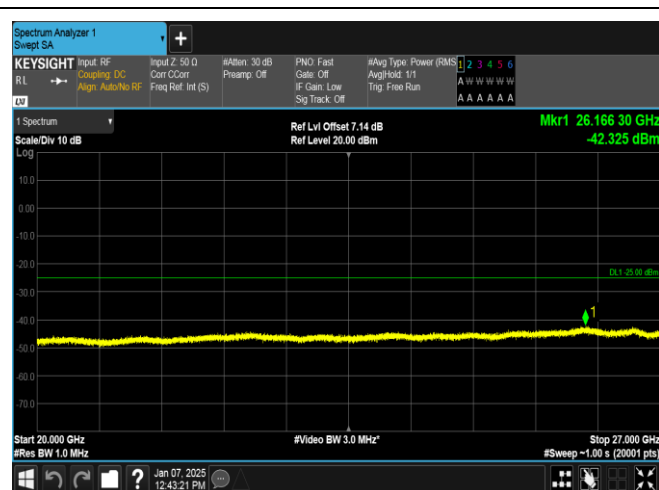
Band7-15MHz-QPSK-20825-1RB#74-20000~27000-PASS
