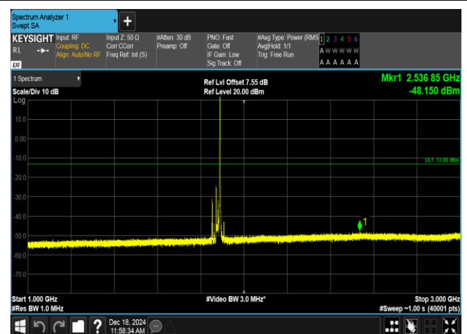
Band2-20MHz-QPSK-18900-1RB#99-1000~3000-PASS
