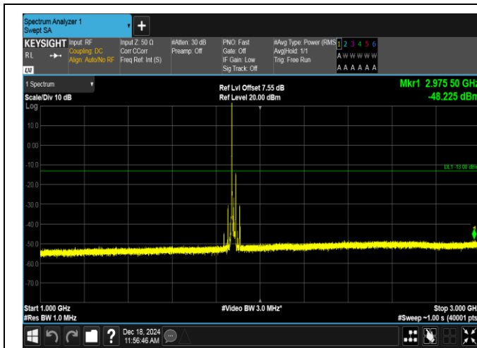
Band2-20MHz-QPSK-18900-1RB#0-1000~3000-PASS
