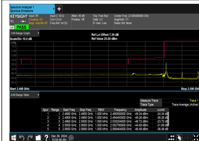
Band38-20MHz-QPSK-37850-1RB#0-PASS
