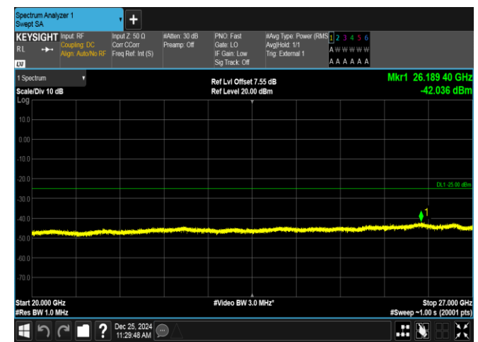
Band38-5MHz-QPSK-38000-25RB#0-20000~27000-PASS
