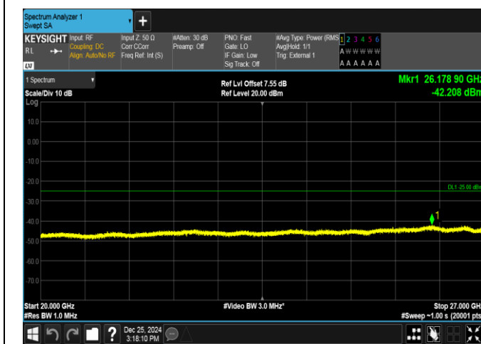
Band38-15MHz-QPSK-37825-1RB#0-20000~27000-PASS
