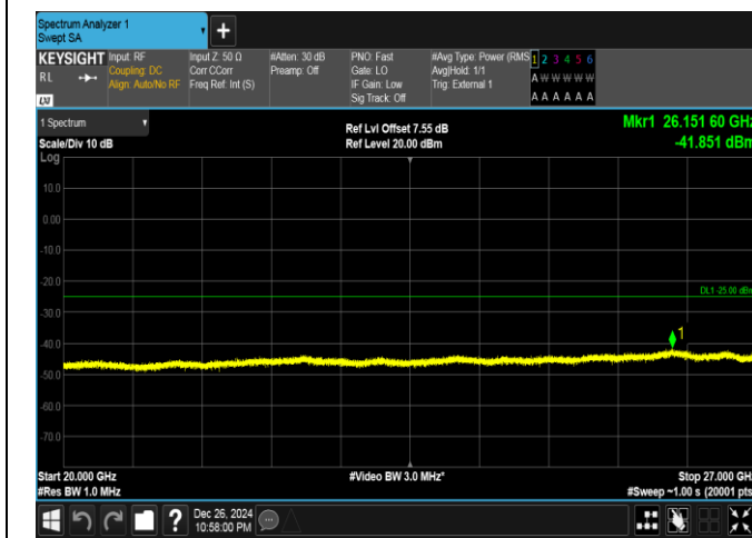
Band41-15MHz-QPSK-39725-1RB#0-20000~27000-PASS
