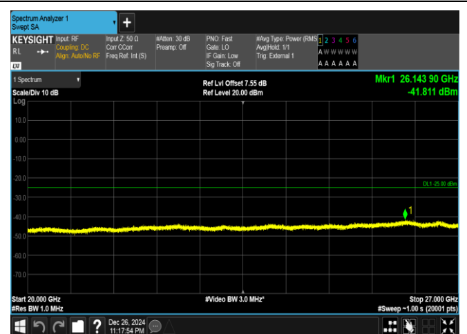
Band41-15MHz-16QAM-41515-1RB#0-20000~27000-PASS
