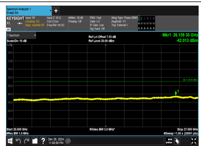
Band41-15MHz-QPSK-39725-1RB#74-20000~27000-PASS
