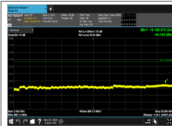
Band66-20MHz-QPSK-132072-100RB#0-3000~20000-PAS
