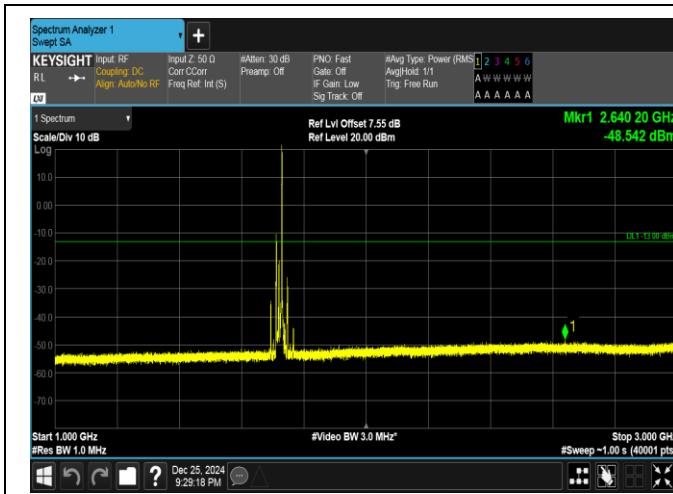
Band66-20MHz-QPSK-132072-1RB#99-1000~3000-PASS
