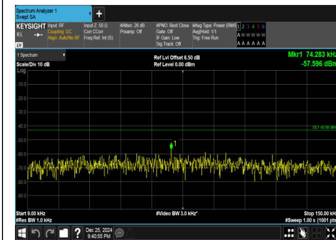
Band66-20MHz-QPSK-132572-1RB#0-0.009~0.15-PASS
