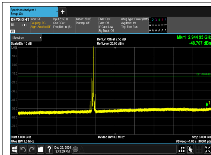
Band66-20MHz-QPSK-132572-1RB#99-1000~3000-PASS
