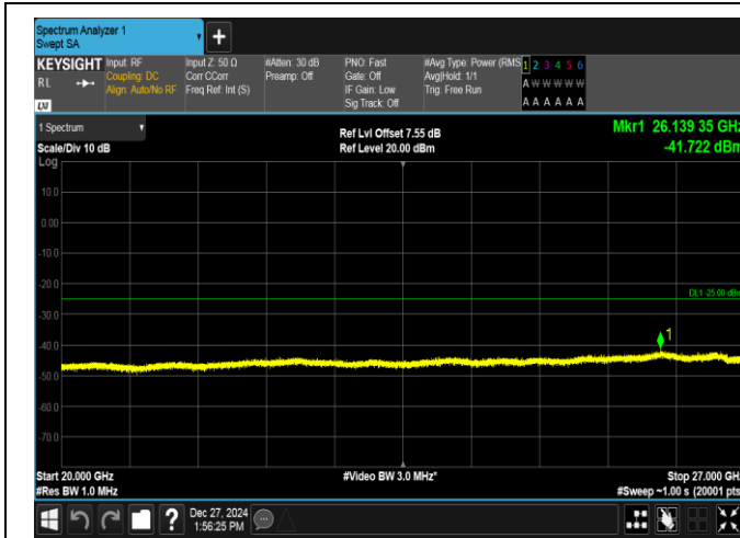
Band7-20MHz-QPSK-20850-100RB#0-20000~27000-PASS
