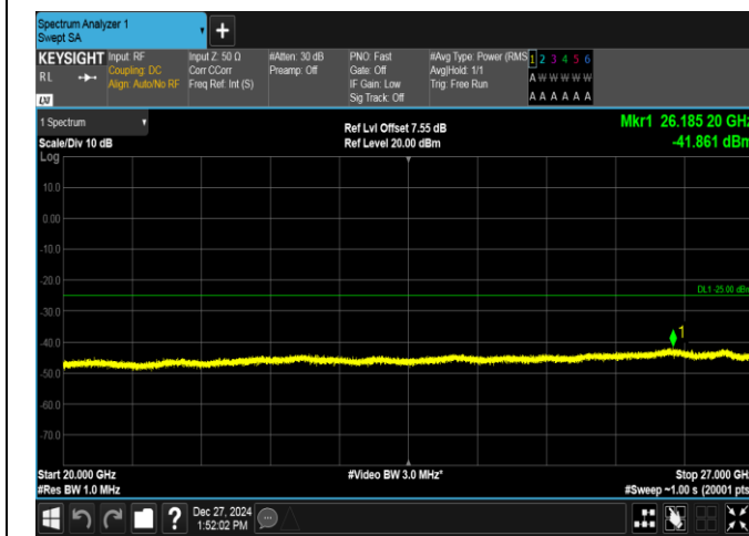
Band7-20MHz-QPSK-20850-1RB#0-20000~27000-PASS
