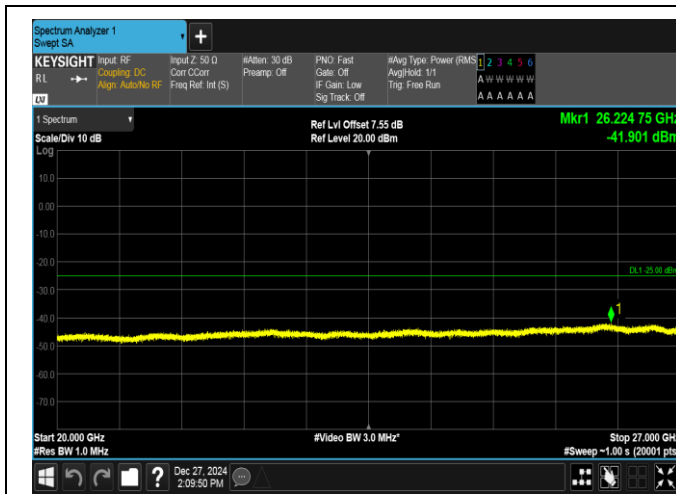
Band7-20MHz-QPSK-21350-100RB#0-20000~27000-PASS
