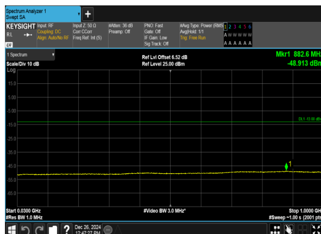
Band2-9538-3-30~1000MHz-PASS
