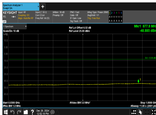
Band2-9538-5-30~1000MHz-PASS
