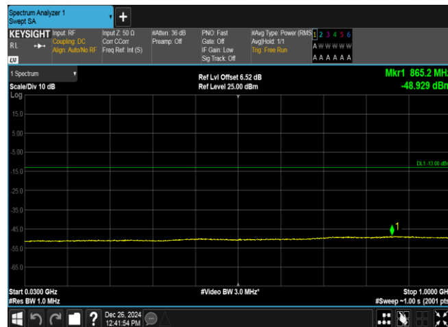
Band2-9400-1-30~1000MHz-PASS
