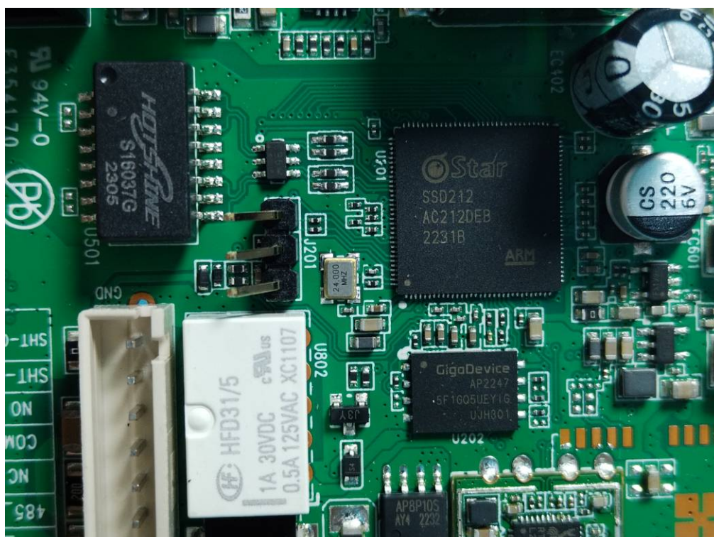
IC Chip 2
