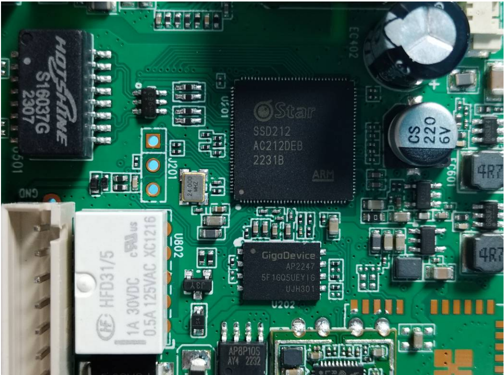
IC Chip 1
