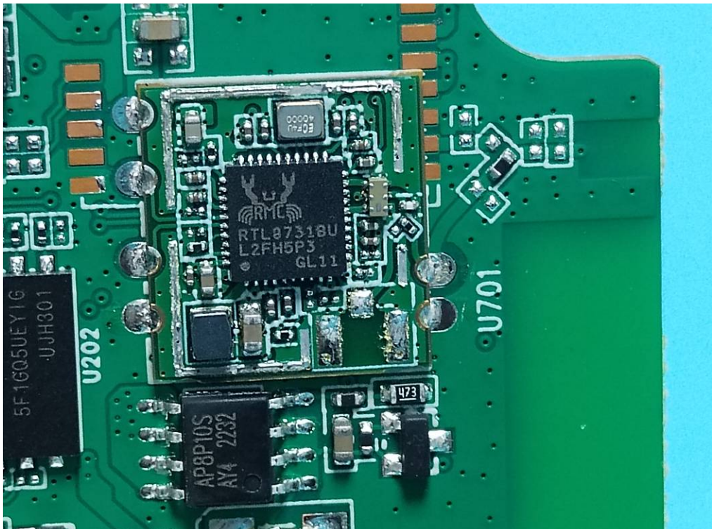
IC Chip 2
