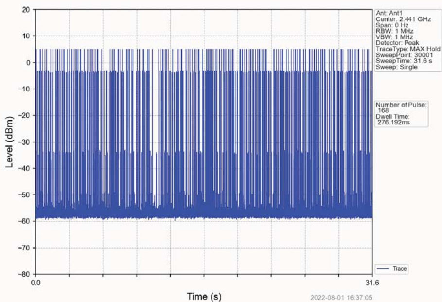
GFSK_DH3_HOPP_Ant1_NTNV
