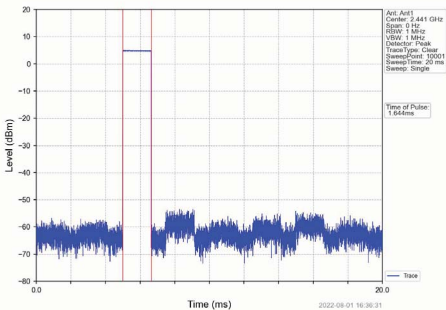
GFSK_DH3_HOPP_Ant1_NTNV
