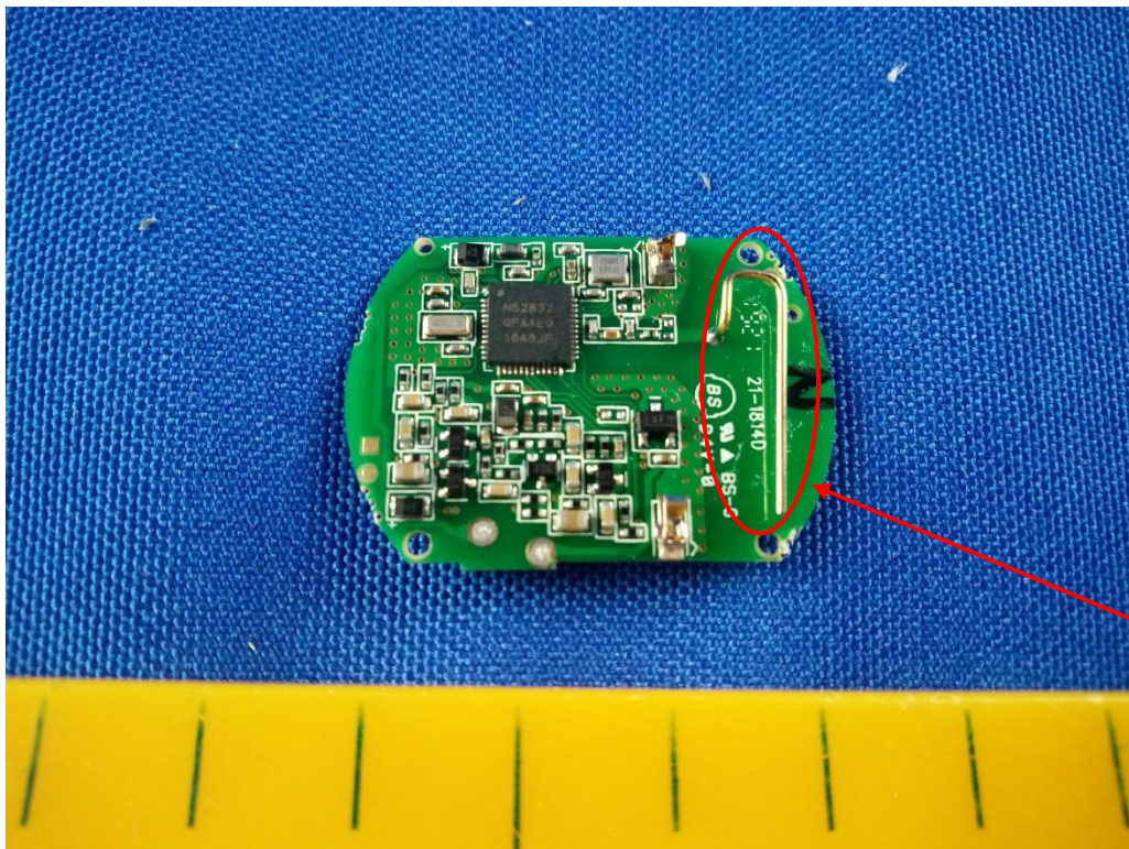
2.4G Antenna
