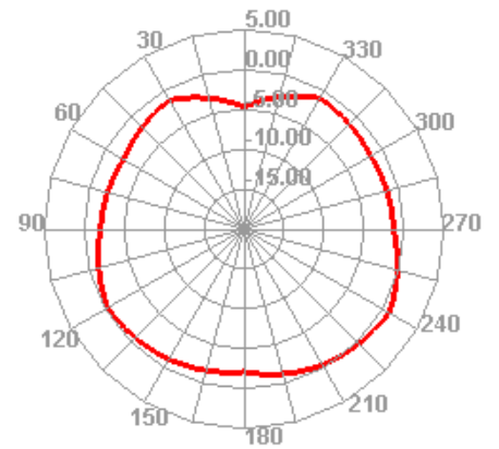
5825MHz E1
