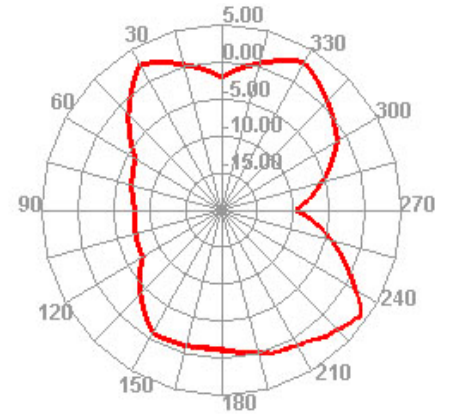
5825MHz H
