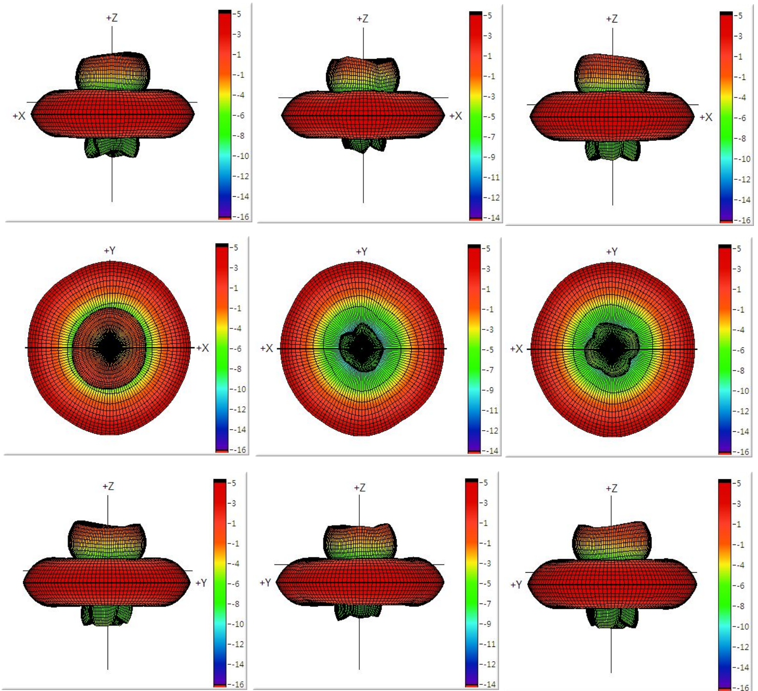
2450MHz
