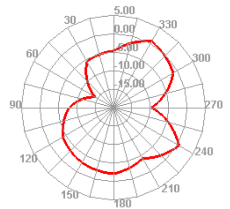
5825MHz E2
