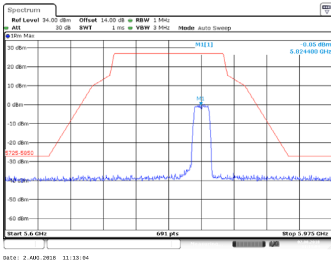
ANT 1(11AC) 5825MHz
