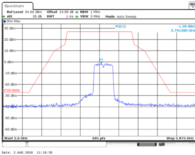
ANT 1(11AC) 5795MHz
