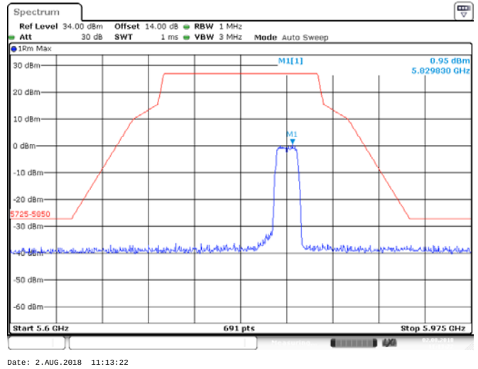
ANT 2(11AC) 5825MHz
