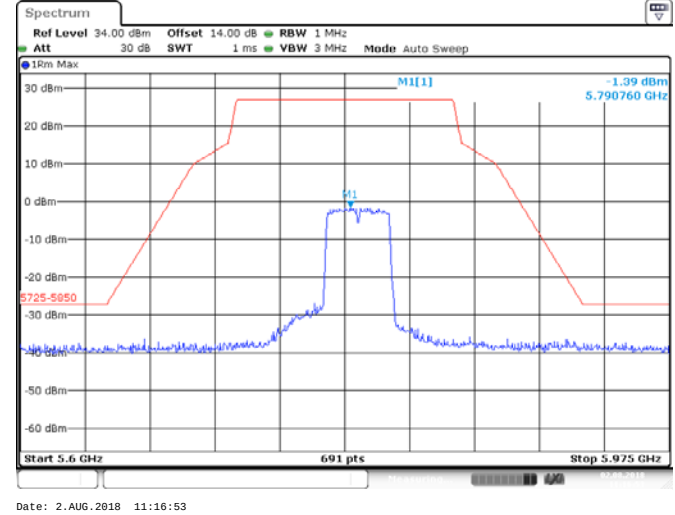
ANT 2(11AC) 5795MHz
