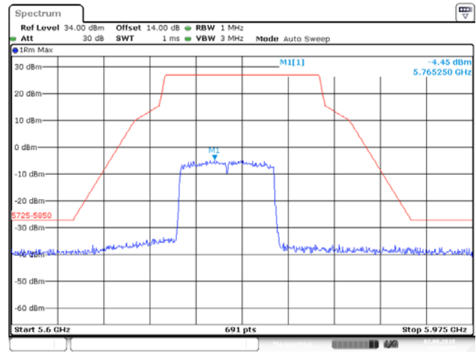
ANT 2(11AC) 5775MHz
