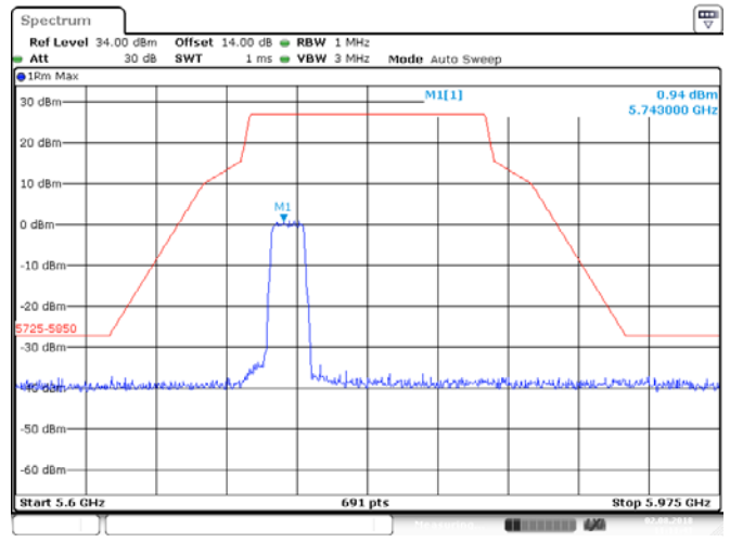
ANT 2(11AC) 5745MHz
