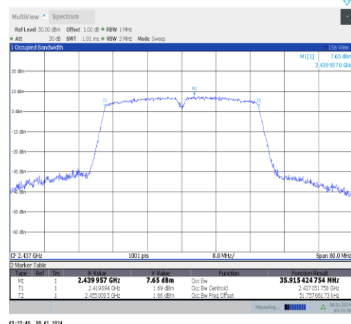
11n40MIMO-Ant1-2437
