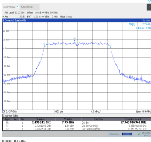
11n20MIMO-Ant0-2437
