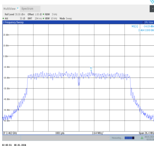
11n20MIMO-Ant0-2462-PASS
