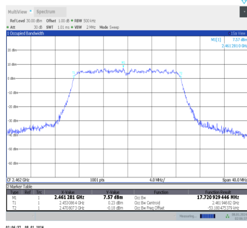
11n20MIMO-Ant1-2462
