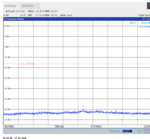
11g-Ant1-2437-30~1000-PASS
