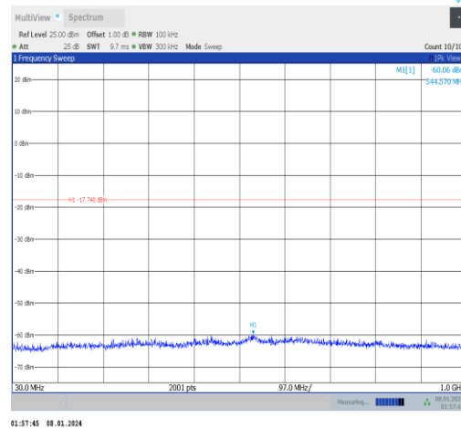
11n20MIMO-Ant0-2412-30~1000-PASS
