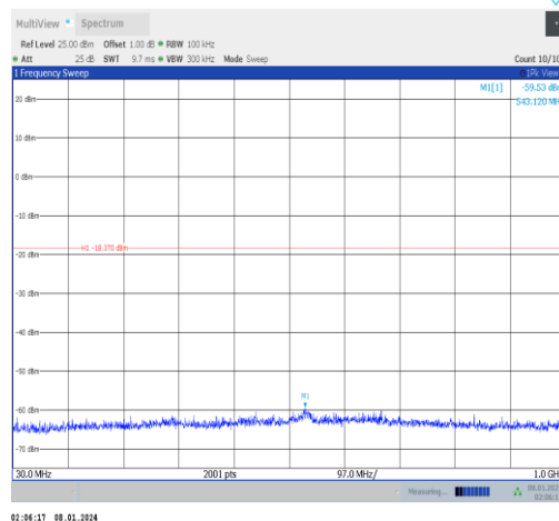
11n20MIMO-Ant0-2462-30~1000-PASS
