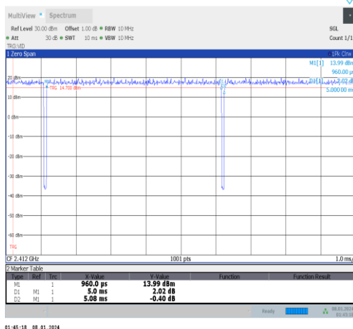
NTNV-11n20MIMO-Ant0-2412
