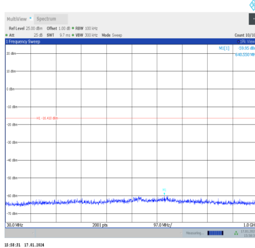
11g-Ant1-2412-30~1000-PASS
