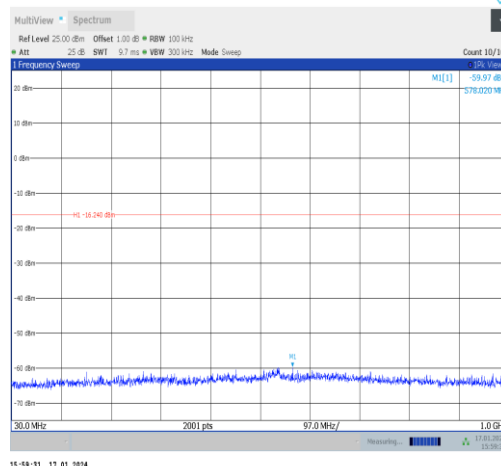
11g-Ant1-2462-30~1000-PASS
