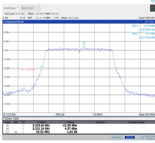
11ac20MIMO-Ant1-5220
