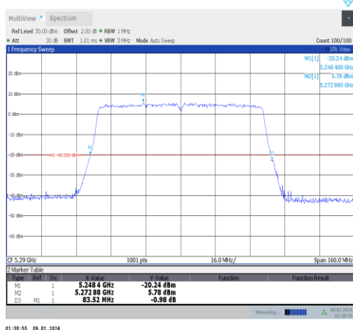
11ac80MIMO-Ant1-5290
