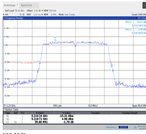
11ac40MIMO-Ant0-5230
