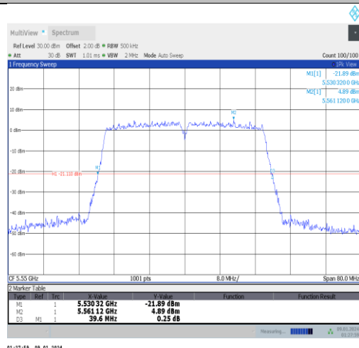
11ac40MIMO-Ant0-5550
