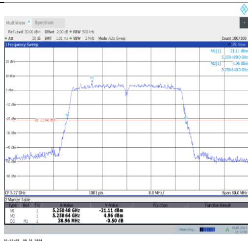
11ac40MIMO-Ant1-5270
