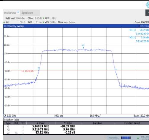
11ac80MIMO-Ant0-5210
