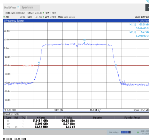
11ac80MIMO-Ant0-5290
