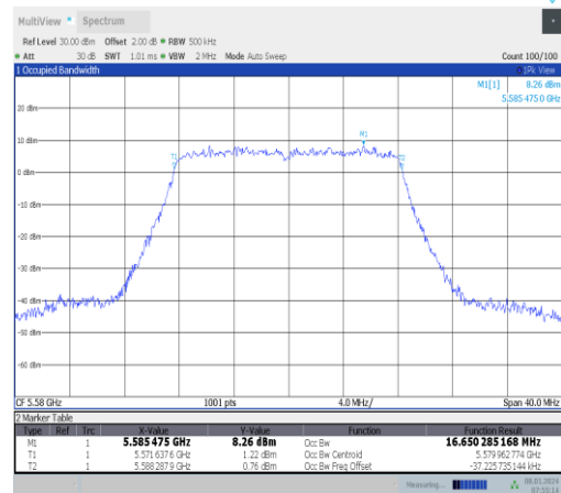
11a-Ant0-5580
