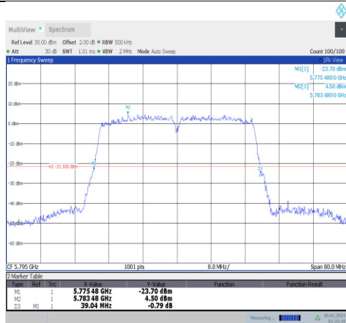
11ac40MIMO-Ant1-5795
