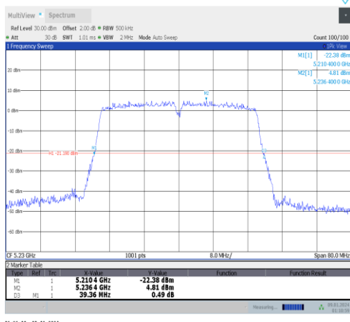
11ac40MIMO-Ant1-5230
