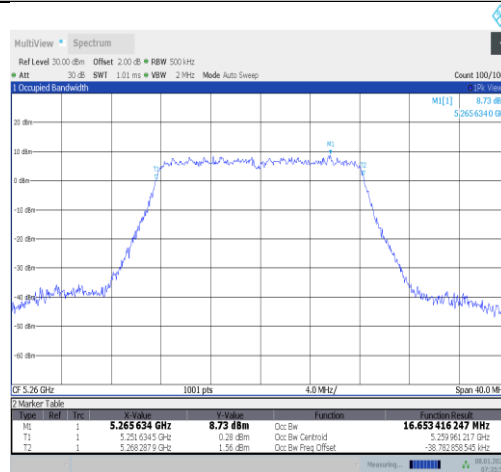
11a-Ant0-5260
