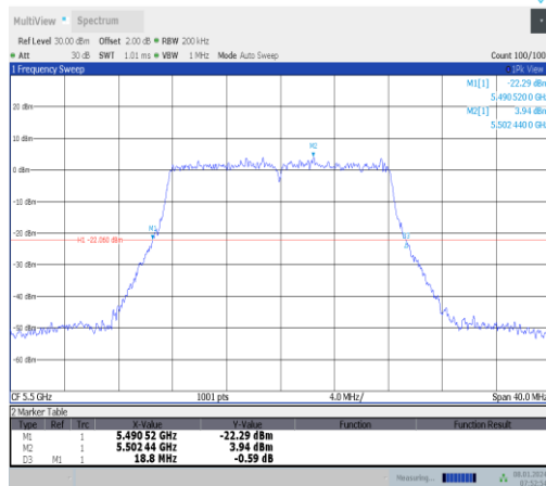
11a-Ant0-5500
