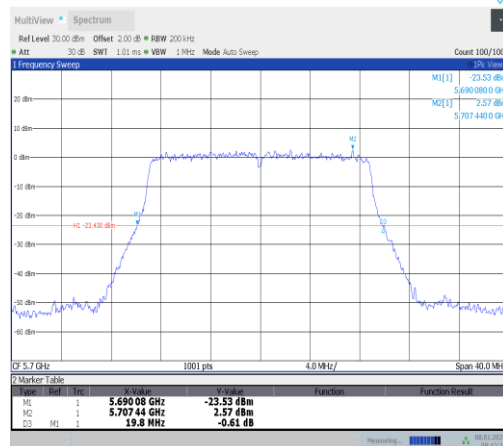
11ac20MIMO-Ant0-5700
