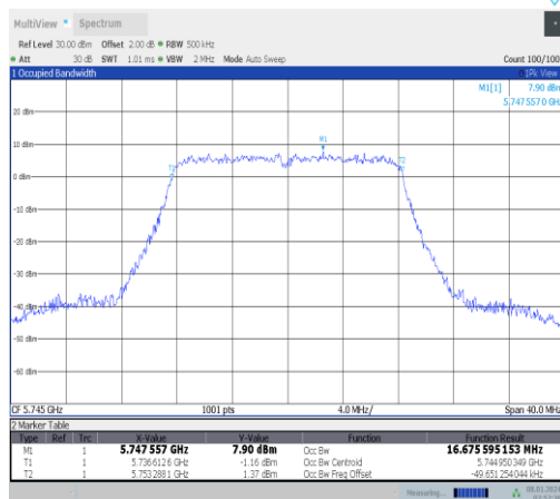
11a-Ant0-5745
