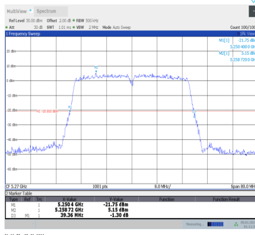
11ac40MIMO-Ant0-5270
