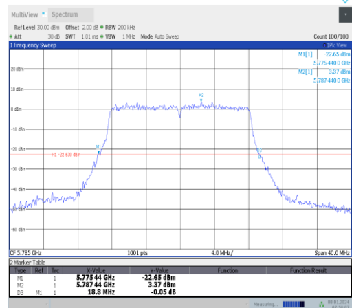
11a-Ant0-5785
