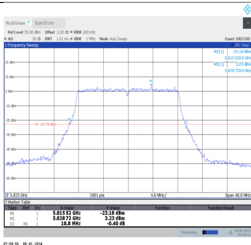
11a-Ant0-5825
