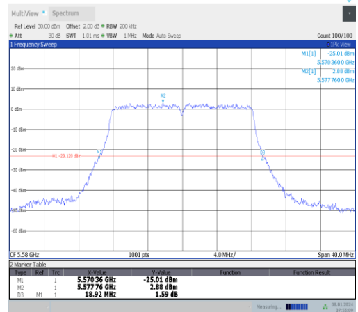
11a-Ant0-5580
