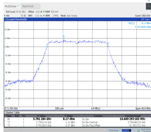
11a-Ant0-5785
