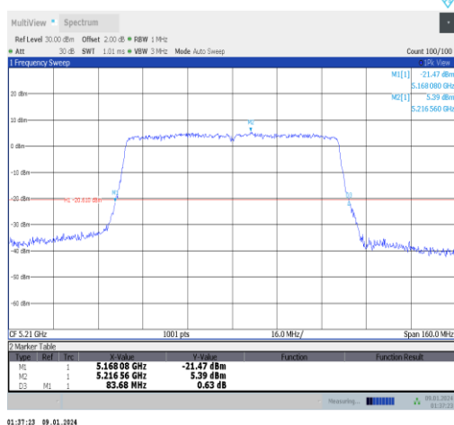
11ac80MIMO-Ant1-5210
