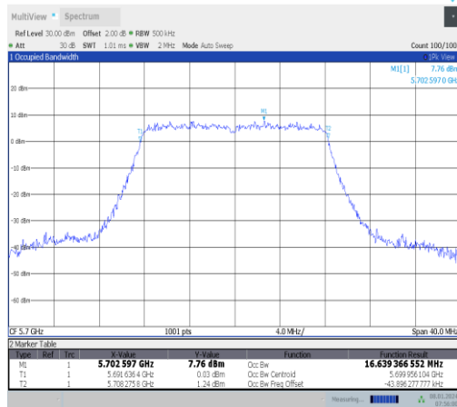
11a-Ant0-5700
