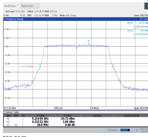
11ac20MIMO-Ant0-5220
