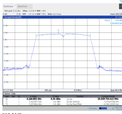
11ac40MIMO-Ant0-5270
