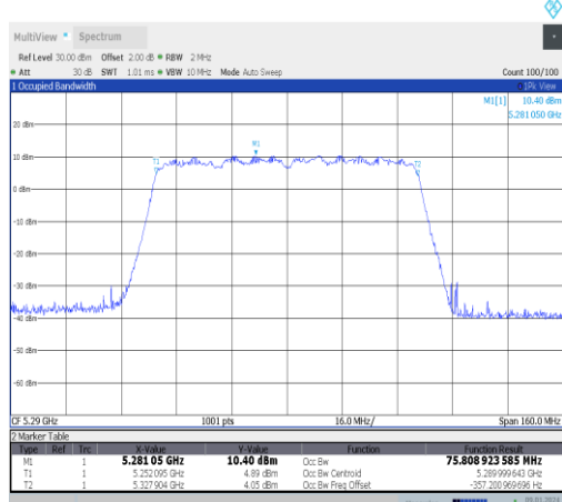
11ac80MIMO-Ant1-5290
