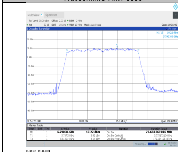
11ac80MIMO-Ant1-5775
