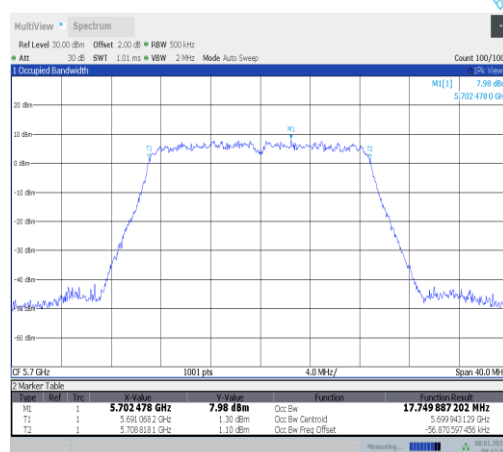
11ac20MIMO-Ant0-5700
