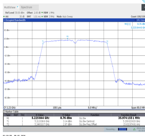
11ac40MIMO-Ant0-5230
