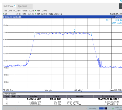
11ac80MIMO-Ant0-5290
