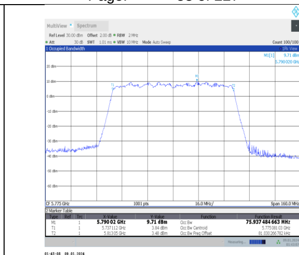
11ac80MIMO-Ant0-5775
