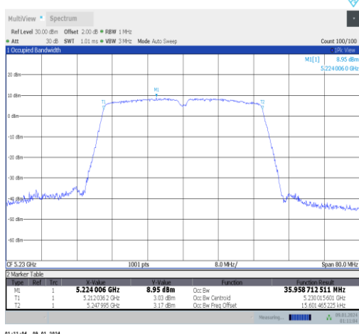
11ac40MIMO-Ant1-5230
