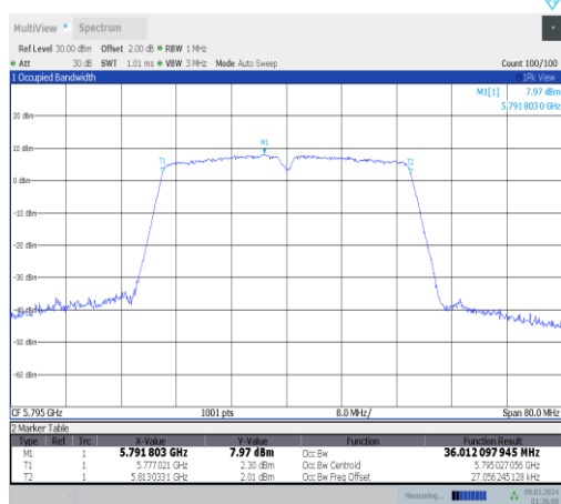
11ac40MIMO-Ant1-5795
