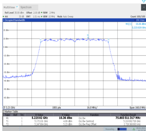
11ac80MIMO-Ant1-5210
