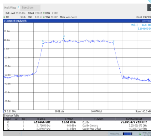
11ac80MIMO-Ant0-5210
