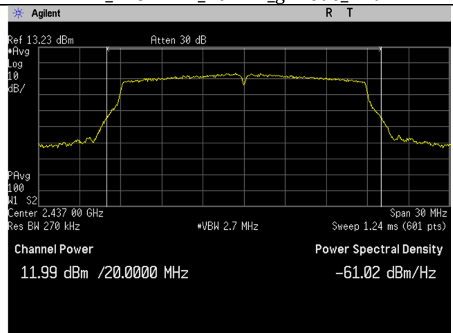
WIFI_2437MHz_20MHz_n-mode_Ant B
