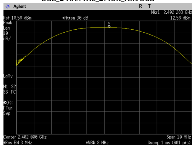
BLE_2402MHz_2MBit_Ant BLE
