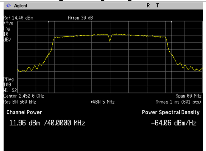
WIFI_2452MHz_40MHz_n-mode_Ant B
