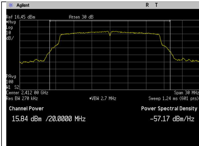
WIFI_2412MHz_20MHz_g-mode_Ant A
