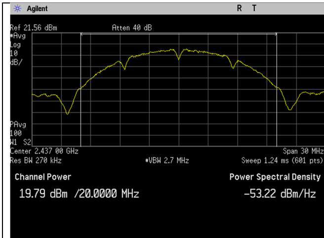
WIFI_2437MHz_20MHz_b-mode_Ant A
