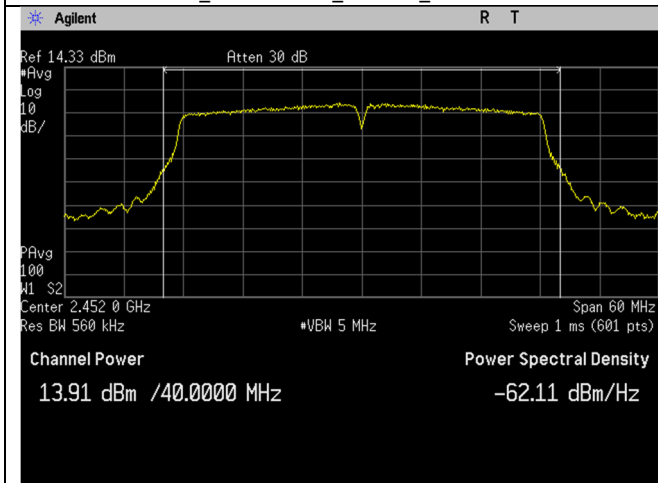
WIFI_2452MHz_40MHz_n-mode_Ant A
