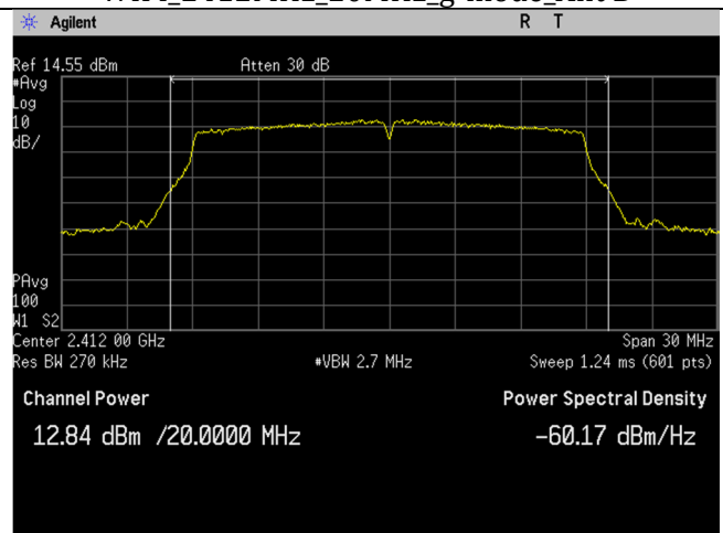
WIFI_2412MHz_20MHz_n-mode_Ant B
