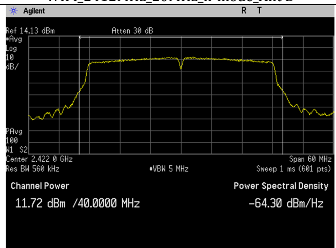
WIFI_2422MHz_40MHz_n-mode_Ant B
