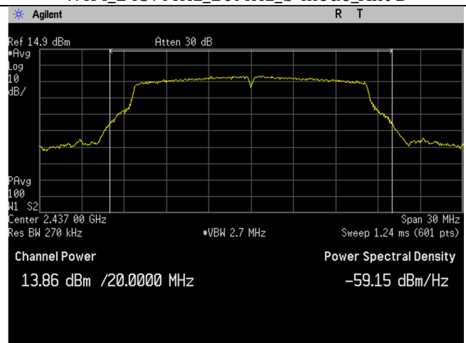
WIFI_2437MHz_20MHz_g-mode_Ant B
