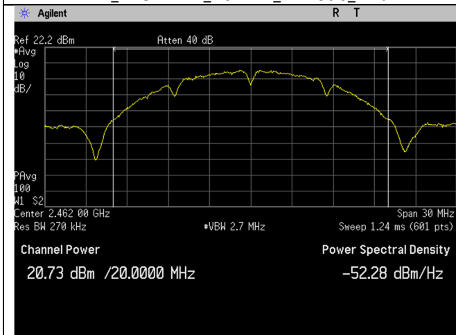
WIFI_2462MHz_20MHz_b-mode_Ant A
