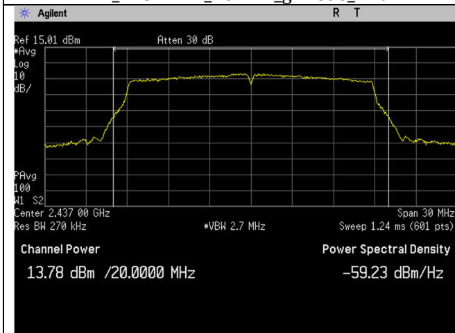
WIFI_2437MHz_20MHz_n-mode_Ant A
