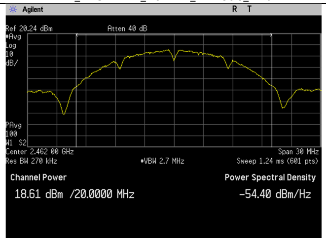
WIFI_2462MHz_20MHz_b-mode_Ant B
