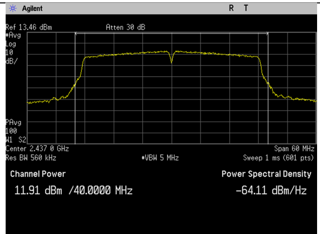
WIFI_2437MHz_40MHz_n-mode_Ant B
