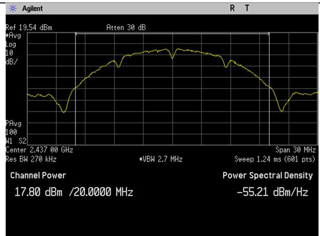
WIFI_2437MHz_20MHz_b-mode_Ant B
