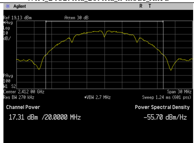
WIFI_2412MHz_20MHz_b-mode_Ant B
