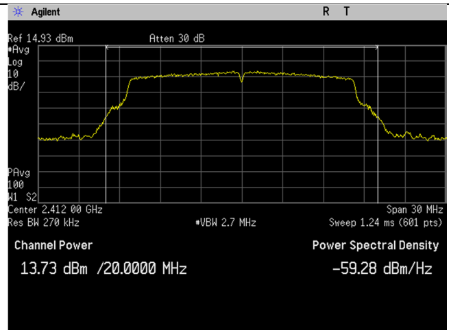
WIFI_2412MHz_20MHz_g-mode_Ant B
