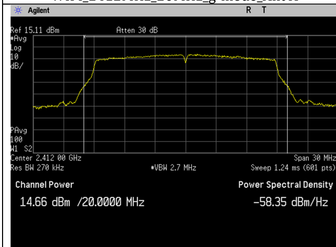
WIFI_2412MHz_20MHz_n-mode_Ant A
