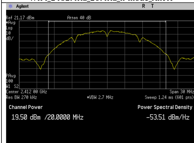
WIFI_2412MHz_20MHz_b-mode_Ant A
