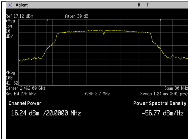
WIFI_2462MHz_20MHz_g-mode_Ant A
