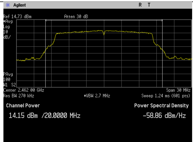
WIFI_2462MHz_20MHz_g-mode_Ant B
