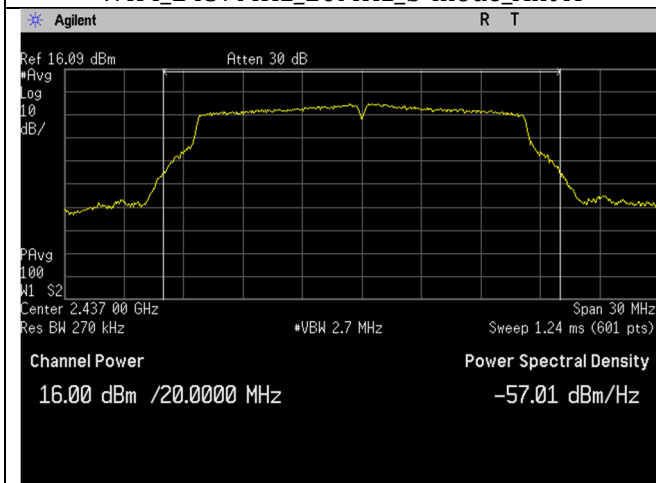
WIFI_2437MHz_20MHz_g-mode_Ant A
