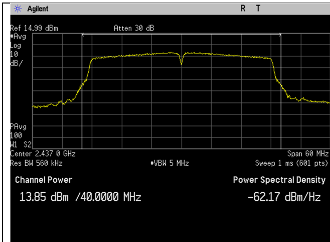
WIFI_2437MHz_40MHz_n-mode_Ant A
