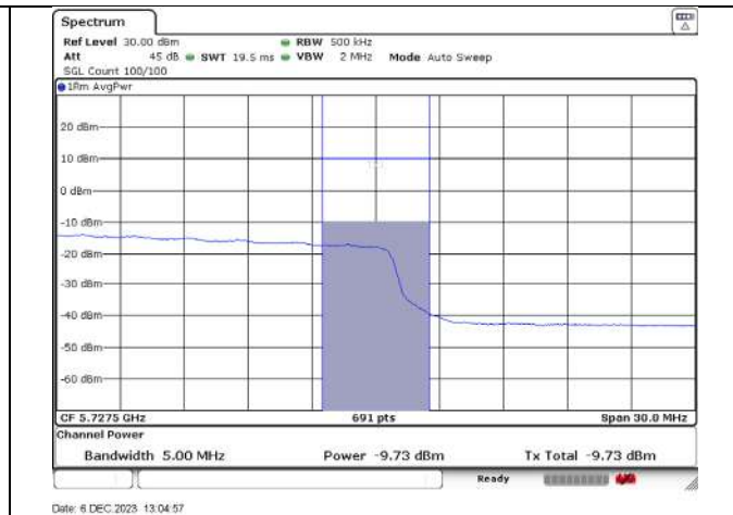
5725-5730MHz_142_40MHz_n-mode_Ant B
