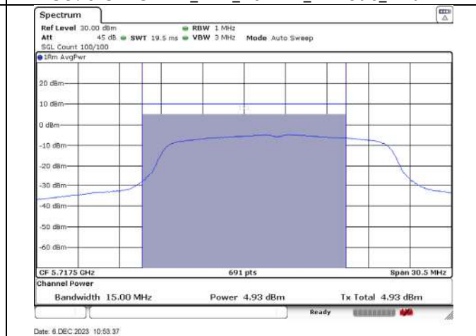
5710-5725MHz_144_20MHz_a-mode_Ant B
