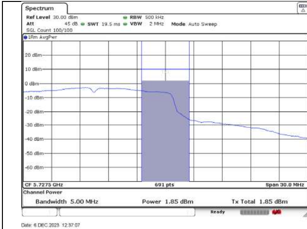
5725-5730MHz_144_20MHz_a-mode_Ant A
