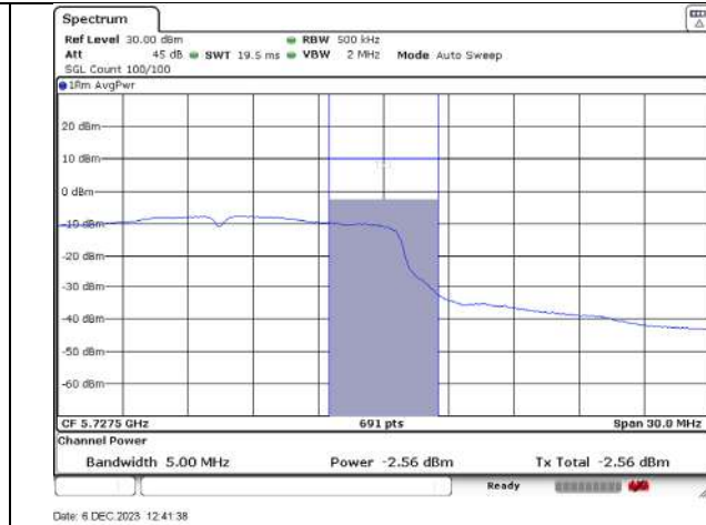
5725-5730MHz_144_20MHz_a-mode_Ant B
