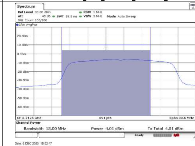
5710-5725MHz_144_20MHz_n-mode_Ant B
