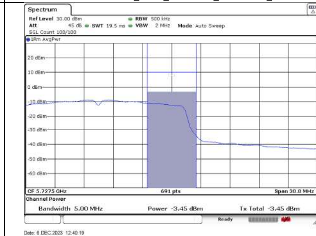
5725-5730MHz_144_20MHz_n-mode_Ant B
