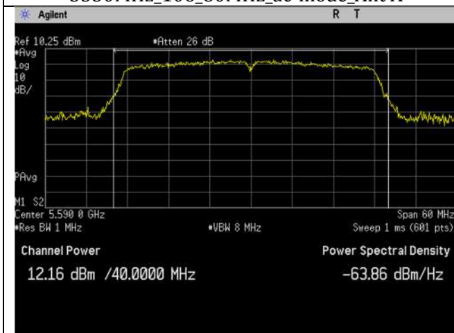
5590MHz_118_40MHz_n-mode_Ant A
