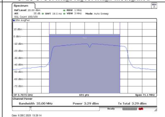
5690-5725MHz_142_40MHz_n-mode_Ant B
