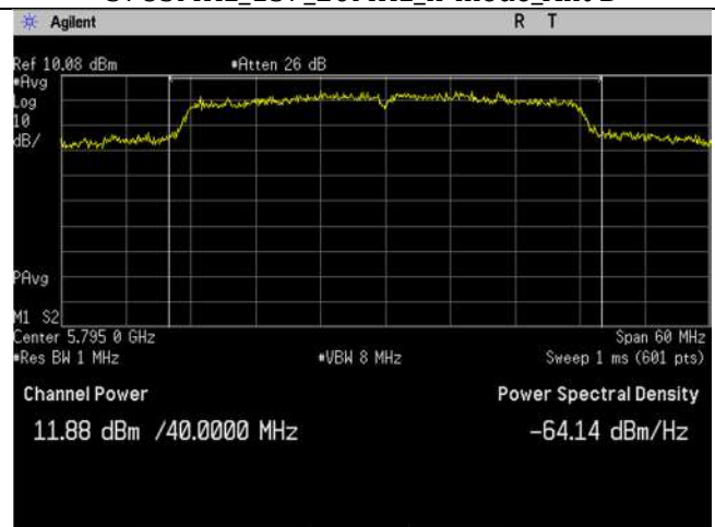
5795MHz_159_40MHz_n-mode_Ant B
