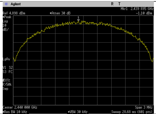
BLE_2440MHz_2MBit_Ant BLE
