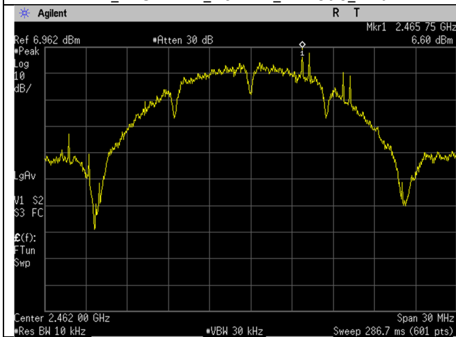
WIFI_2462MHz_20MHz_b-mode_Ant A
