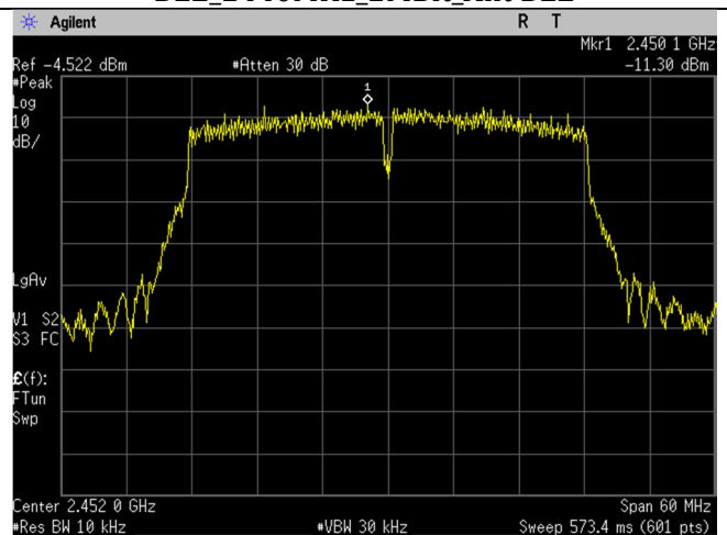
WIFI_2452MHz_40MHz_n-mode_Ant B
