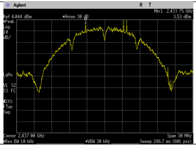
WIFI_2437MHz_20MHz_b-mode_Ant B
