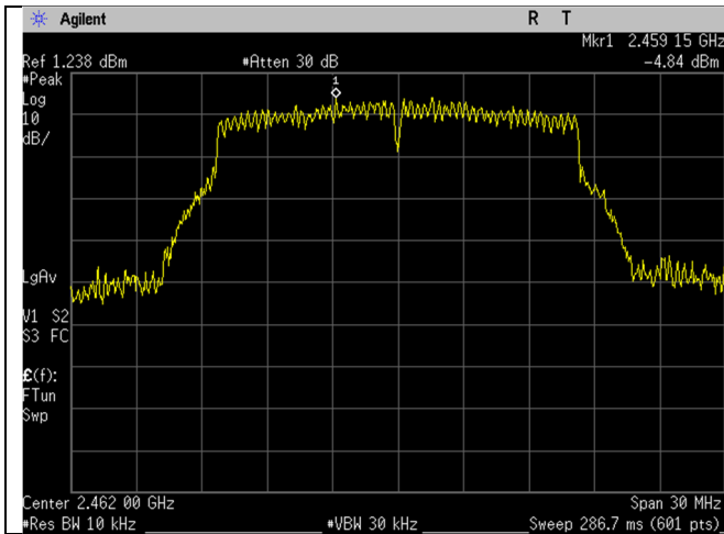
WIFI_2462MHz_20MHz_g-mode_Ant A
