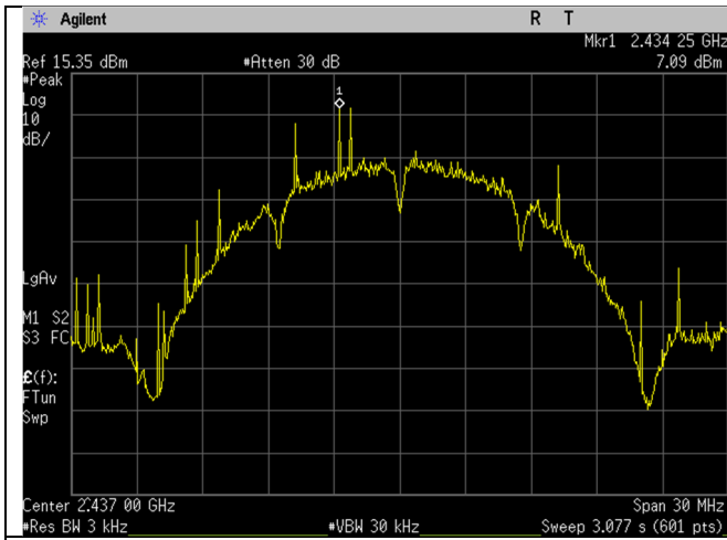
WIFI_2437MHz_20MHz_b-mode_Ant A
