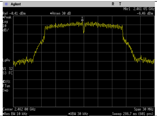
WIFI_2462MHz_20MHz_g-mode_Ant B
