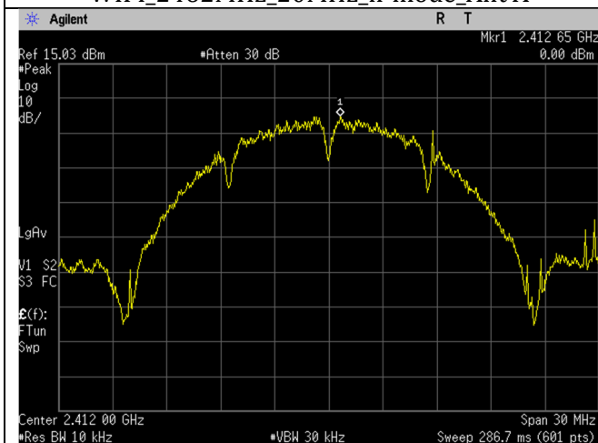
WIFI_2412MHz_20MHz_b-mode_Ant A
