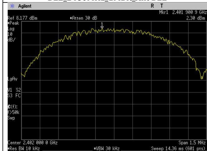
BLE_2402MHz_1MBit_Ant BLE
