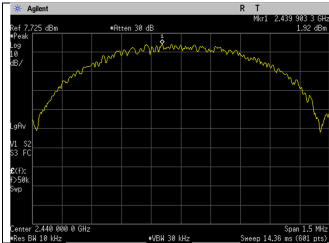
BLE_2440MHz_1MBit_Ant BLE
