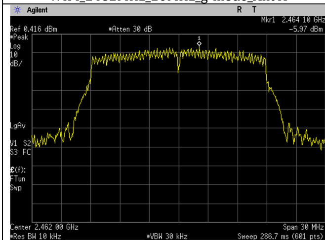
WIFI_2462MHz_20MHz_n-mode_Ant A
