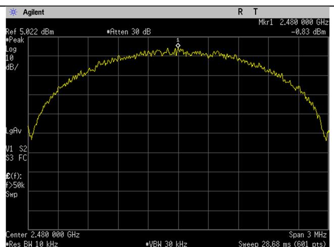
BLE_2480MHz_2MBit_Ant BLE
