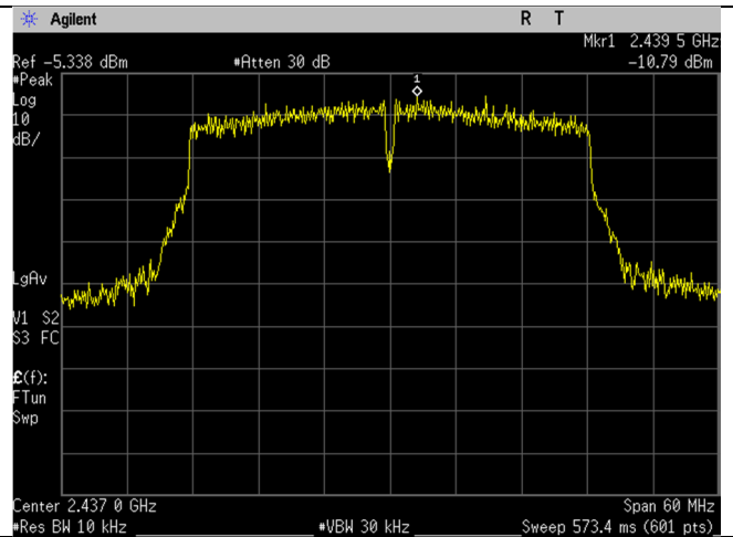
WIFI_2437MHz_40MHz_n-mode_Ant B
