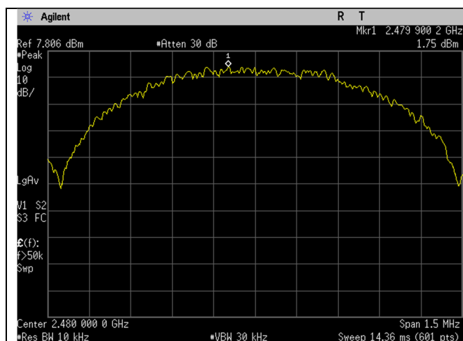
BLE_2480MHz_1MBit_Ant BLE
