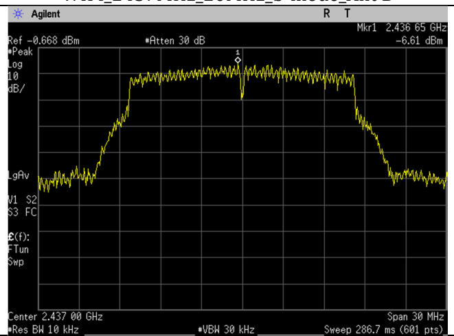
WIFI_2437MHz_20MHz_g-mode_Ant B
