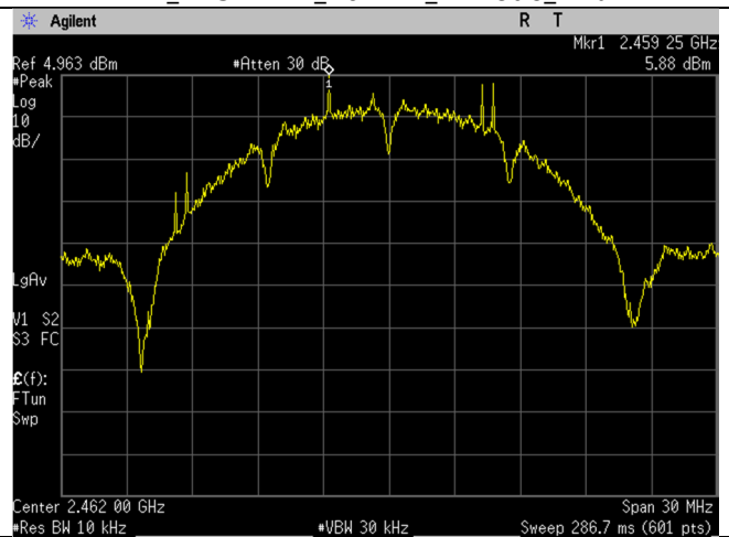
WIFI_2462MHz_20MHz_b-mode_Ant B
