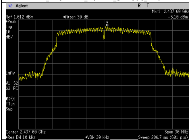
WIFI_2437MHz_20MHz_g-mode_Ant A
