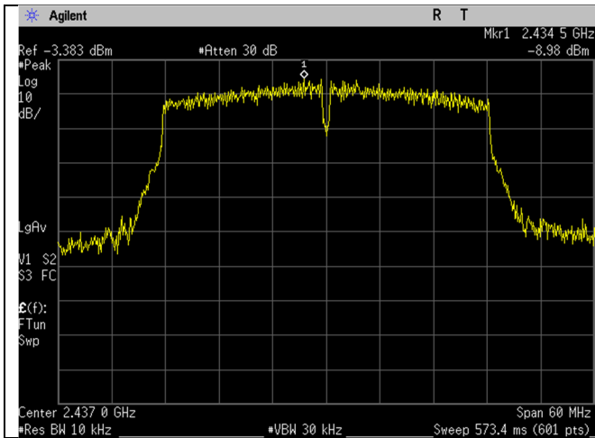
WIFI_2437MHz_40MHz_n-mode_Ant A
