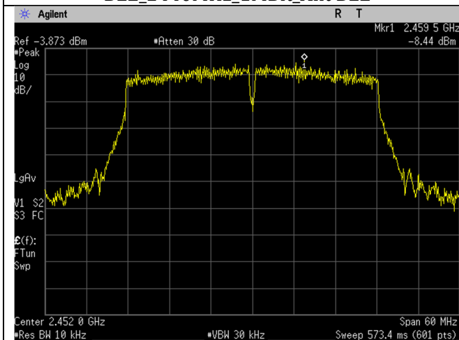
WIFI_2452MHz_40MHz_n-mode_Ant A
