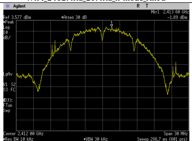
WIFI_2412MHz_20MHz_b-mode_Ant B
