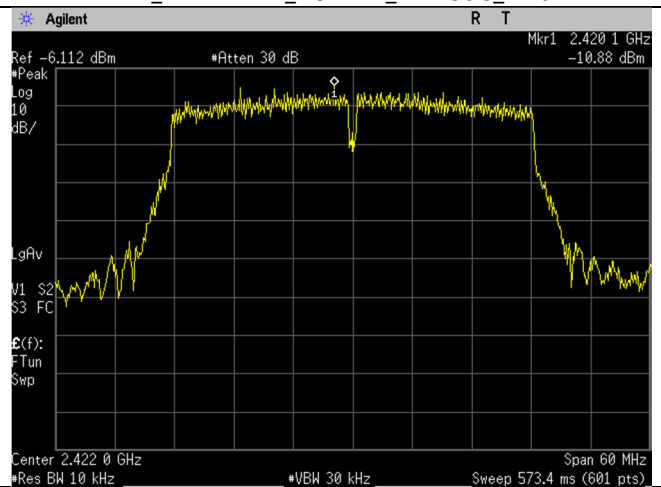
WIFI_2422MHz_40MHz_n-mode_Ant B
