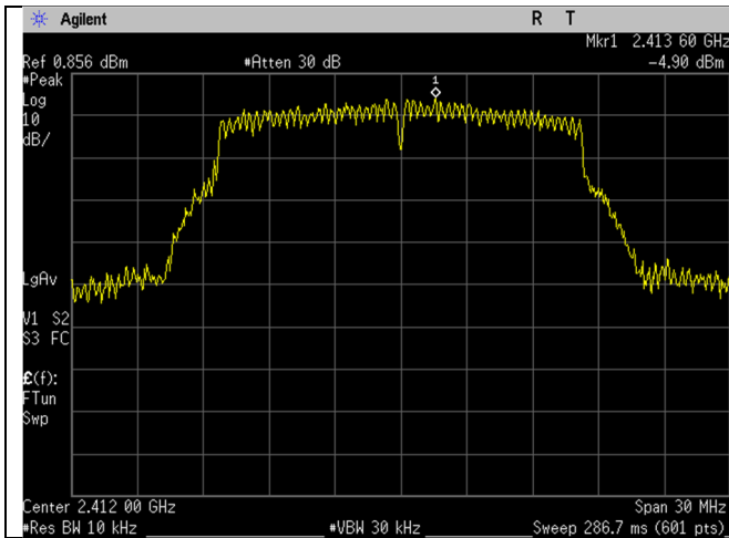
WIFI_2412MHz_20MHz_g-mode_Ant A
