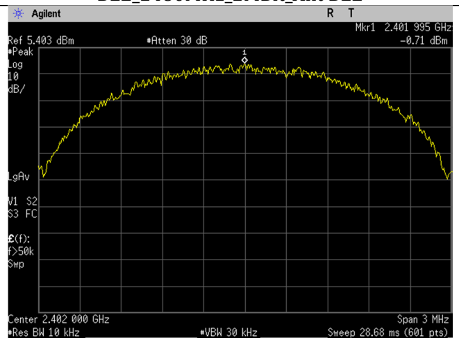
BLE_2402MHz_2MBit_Ant BLE
