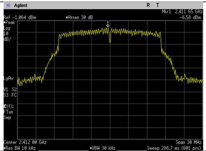
WIFI_2412MHz_20MHz_g-mode_Ant B
