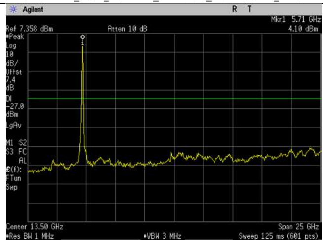
5690MHz_138_80MHz_ac-mode_1-26GHz_Ant B
