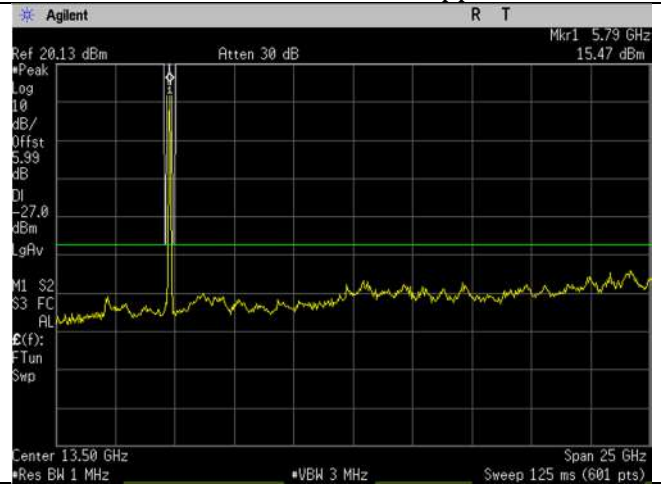
5785MHz_157_20MHz_a-mode_1-26GHz_Ant B
