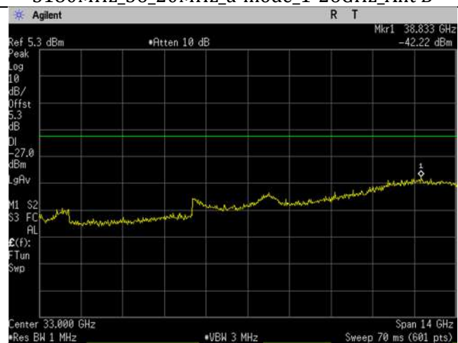
5180MHz_36_20MHz_a-mode_26-40GHz_Ant B
