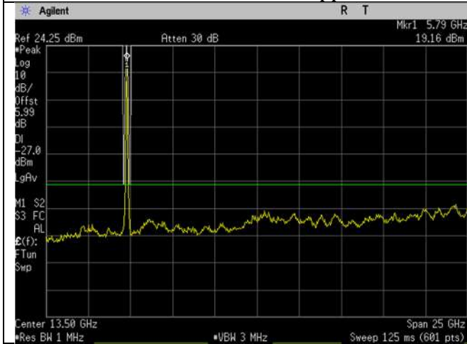
5785MHz_157_20MHz_a-mode_1-26GHz_Ant A
