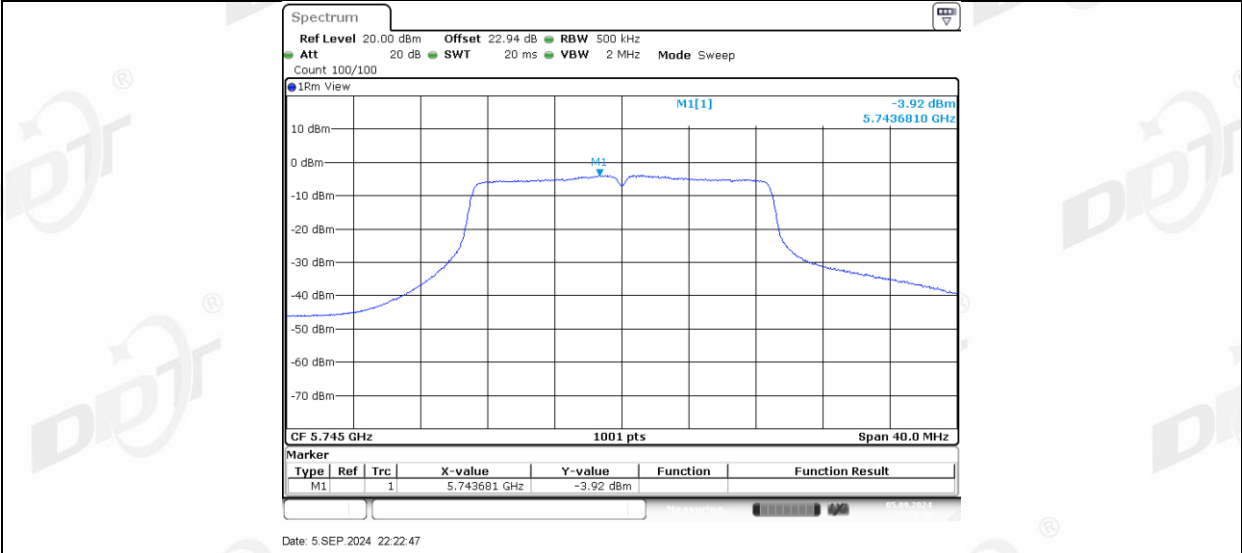
11AC20MIMO_Ant2_5745
