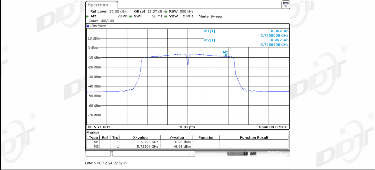
11AC40MIMO_Ant2_5710_UNII-3
