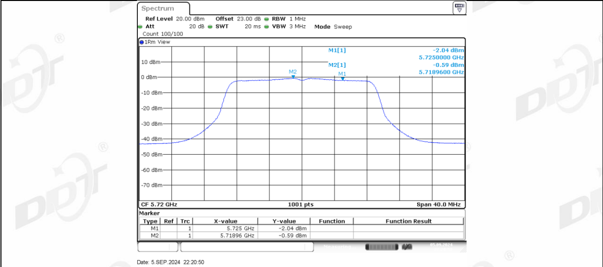
11AC20MIMO_Ant1_5720_UNII-3
