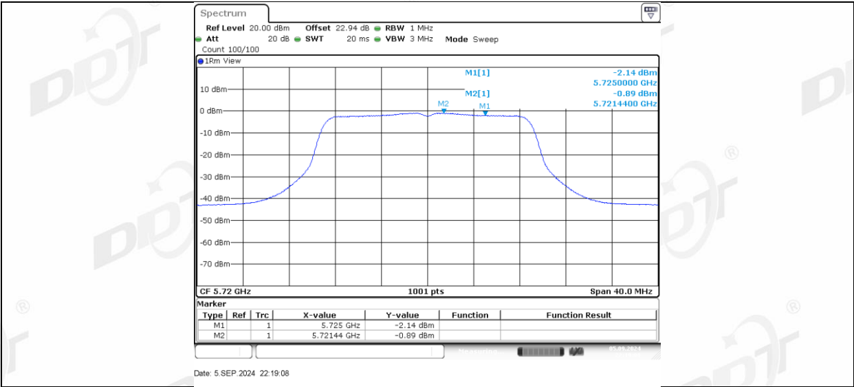
11AC20MIMO_Ant2_5720_UNII-2C
