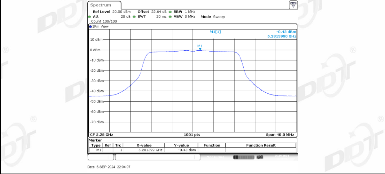
11AC20MIMO_Ant2_5280
