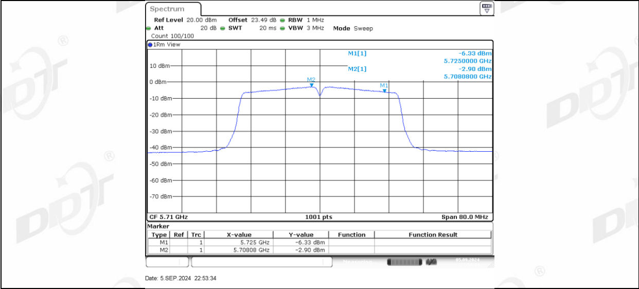
11AC40MIMO_Ant1_5710_UNII-3
