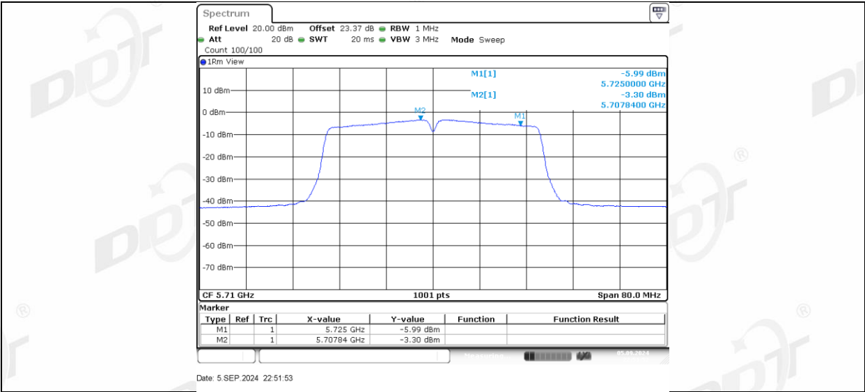
11AC40MIMO_Ant2_5710_UNII-2C
