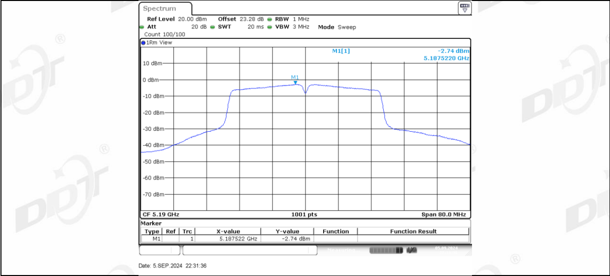
11AC40MIMO_Ant2_5190
