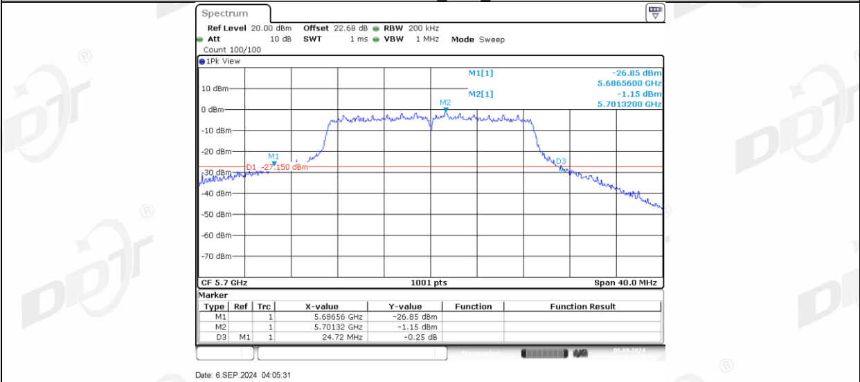
11AC20MIMO_Ant2_5700
