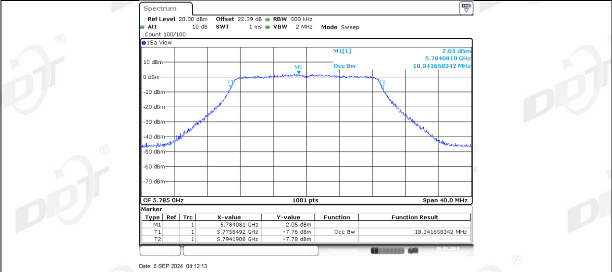
11AC20MIMO_Ant2_5785
