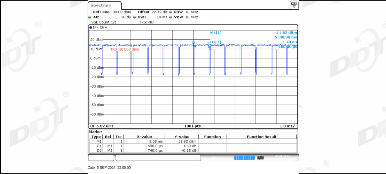
11AC20MIMO_Ant2_5320
