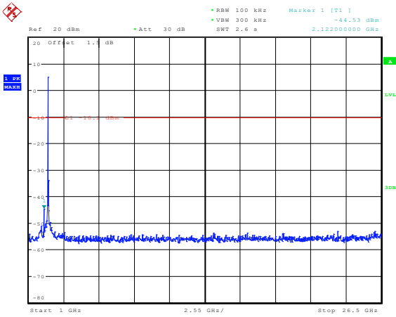
11G ANT1 2437 1000~26500
