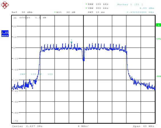
11N40_ANT1_2437_Ref
