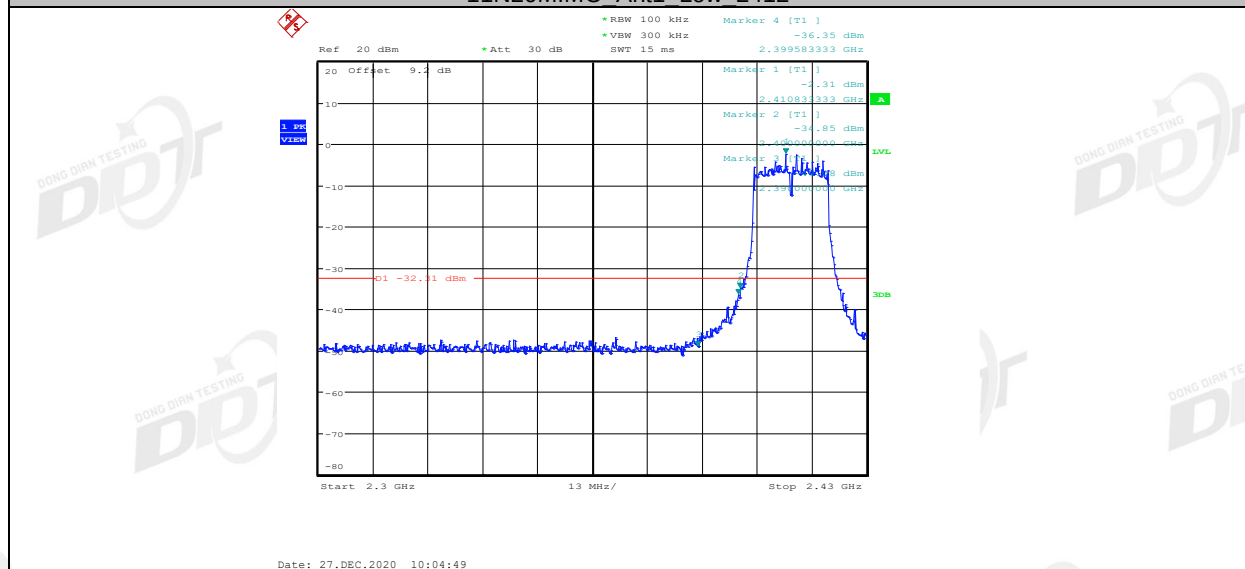
11N20MIMO_Ant2_Low_2412
