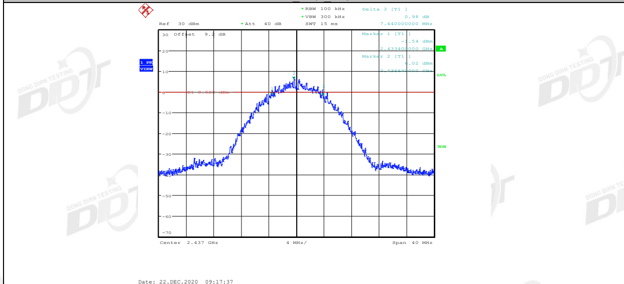
11B Ant2 2437
