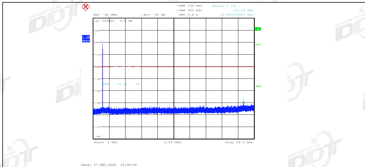
11N40MIMO_Ant1_2422_0-Reference
