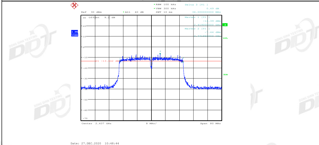
11N40MIMO Ant2 2437
