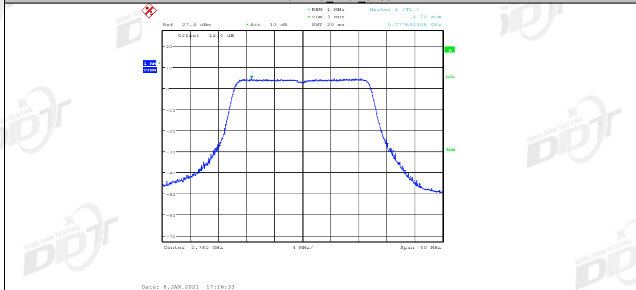
11AX20MIMO Ant2 5785
