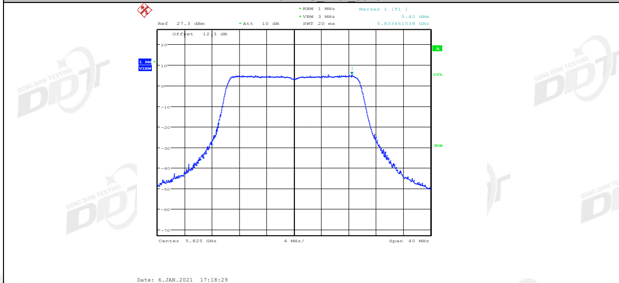
11AX20MIMO_Ant2_5825
