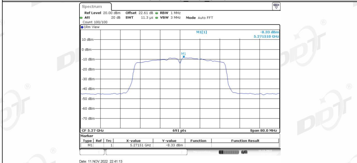
11AC40MIMO_Ant2_5270
