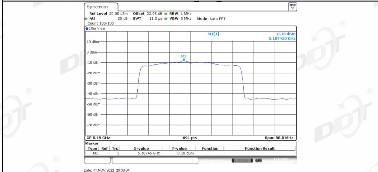
11AX40MIMO_Ant2_5190
