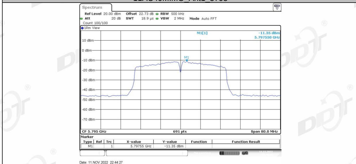
11AC40MIMO_Ant2_5795
