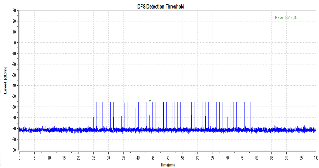
11N40MIMO_5270_Type1
