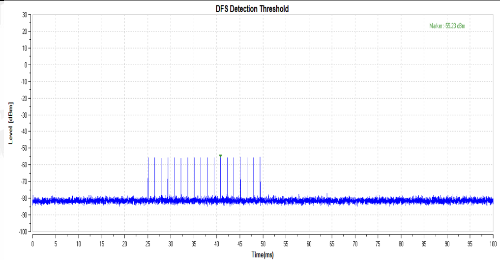
11N40MIMO_5270_Type1
