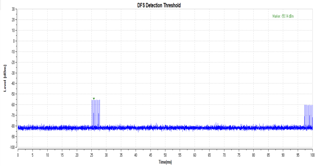
11N40MIMO_5270_Type0
