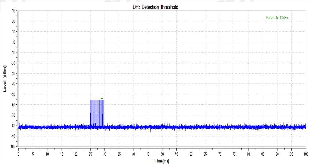
11N40MIMO_5270_Type3
