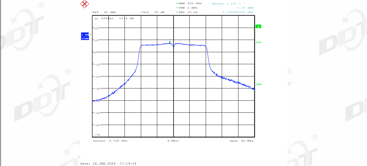
11A_Ant2_5745
