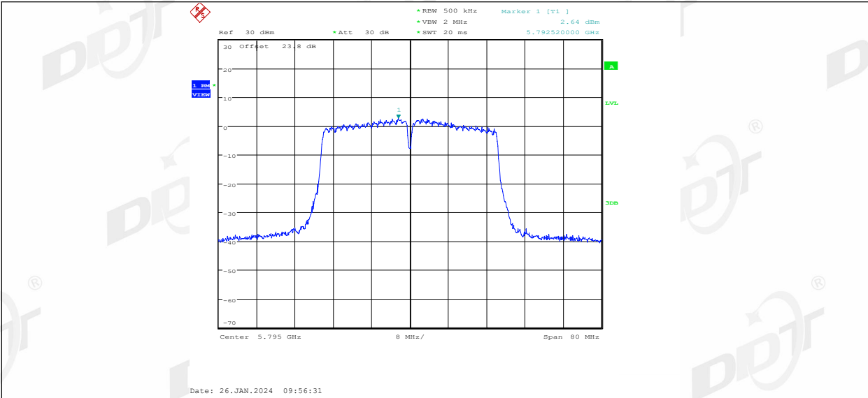
11AC40MIMO_Ant2_5795
