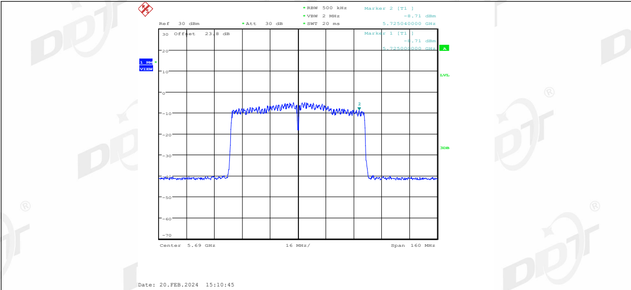
11AC80MIMO_Ant2_5690_UNII-3
