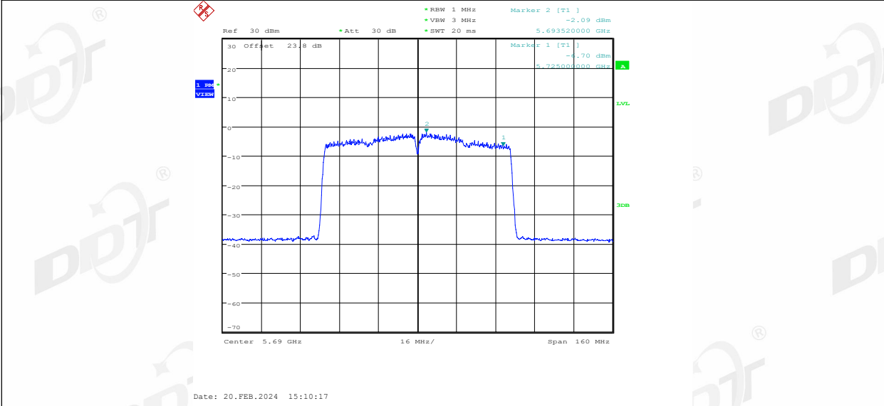
11AC80MIMO_Ant2_5690_UNII-2C
