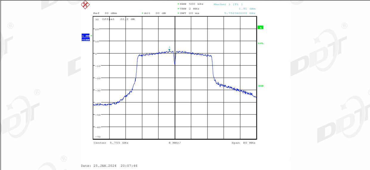
11N40MIMO_Ant2_5755
