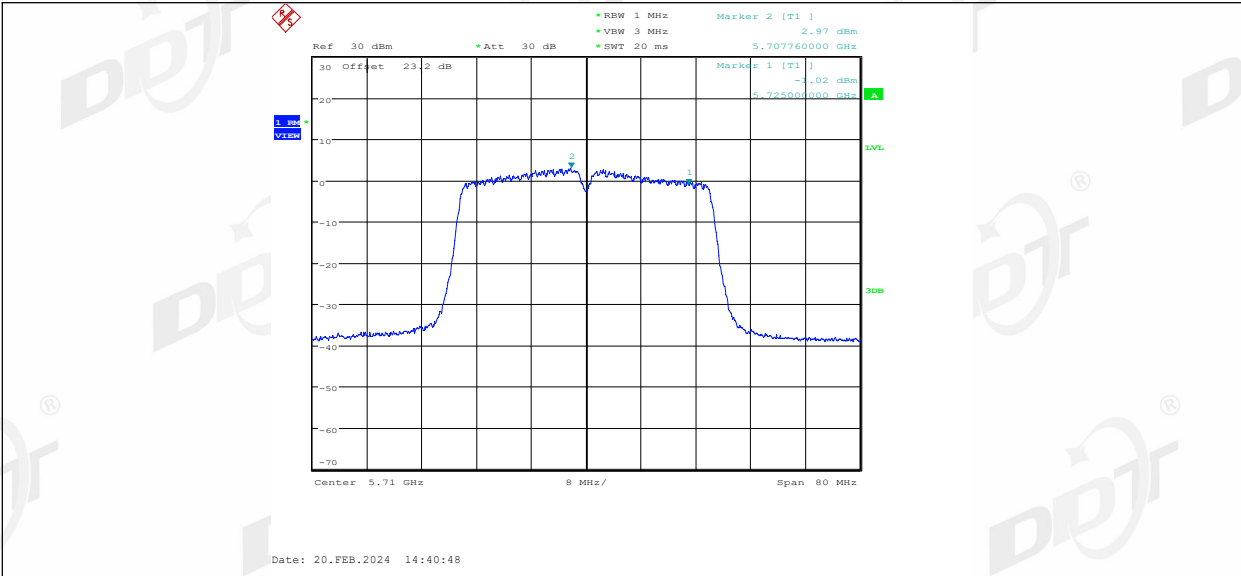
11AC40MIMO_Ant2_5710_UNII-2C
