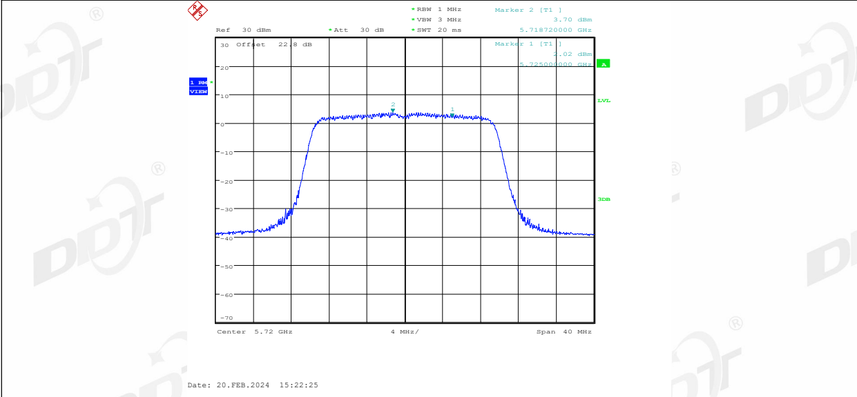
11AX20MIMO_Ant2_5720_UNII-2C
