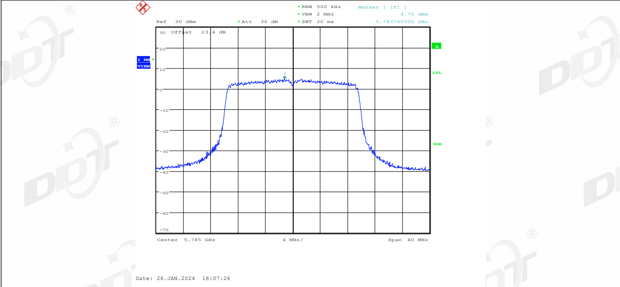
11AX20MIMO_Ant2_5785
