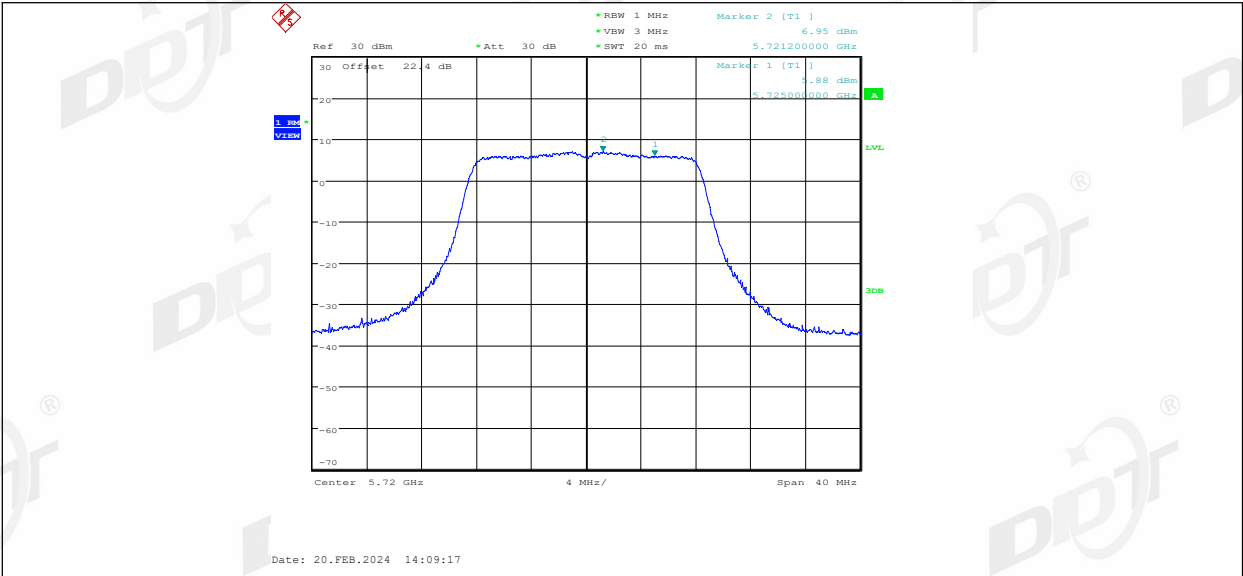
11A_Ant2_5720_UNII-2C
