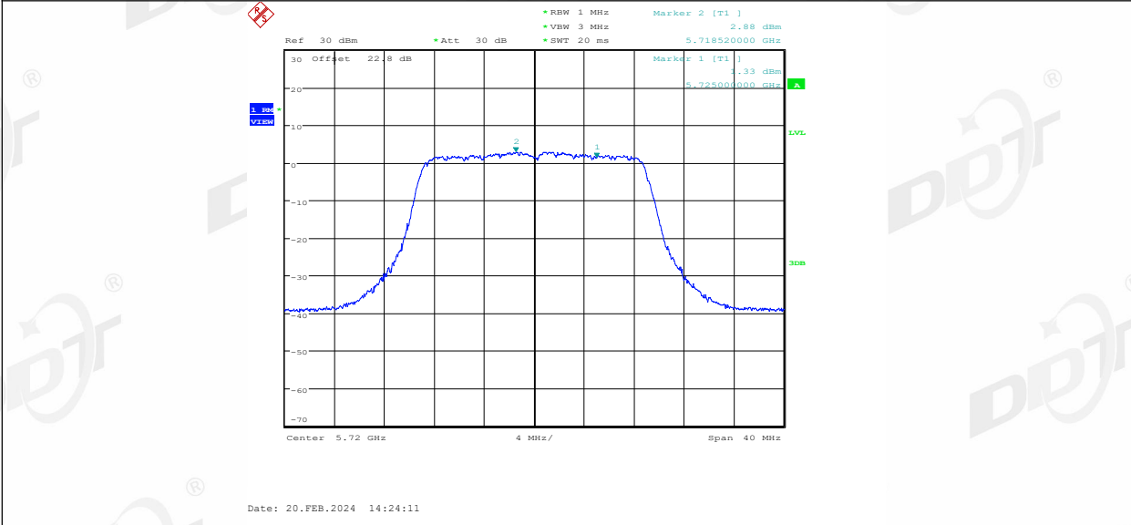
11N20MIMO Ant1_5720_UNII-3
