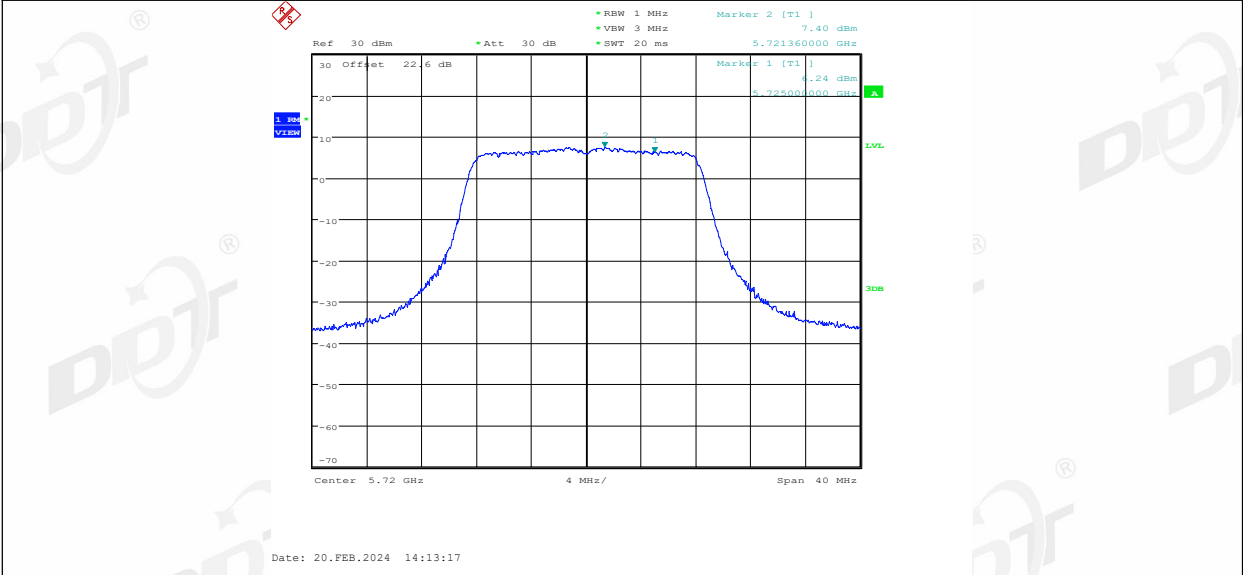
11A_Ant1_5720_UNII-3
