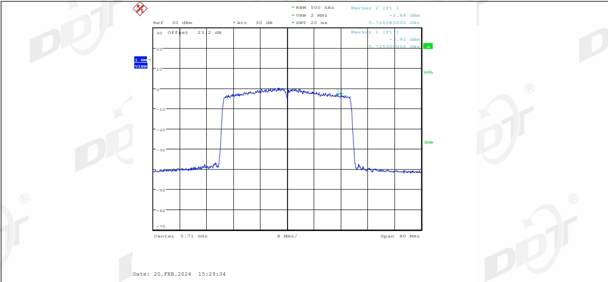
11AX40MIMO_Ant2_5710_UNII-3
