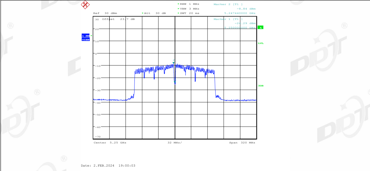
11AC160MIMO_Ant1_5250_UNII-2A
