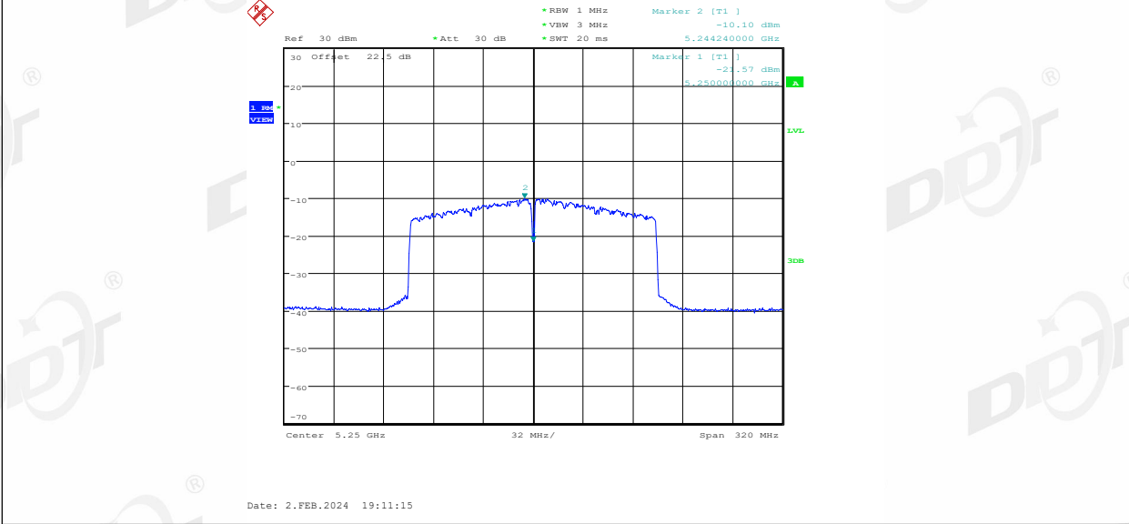
11AX160MIMO_Ant2_5250_UNII-1
