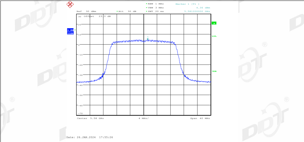
11AX20MIMO_Ant2_5580
