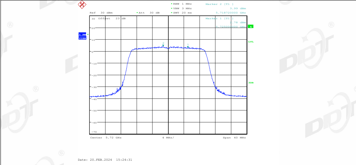
11AX20MIMO_Ant1_5720_UNII-3
