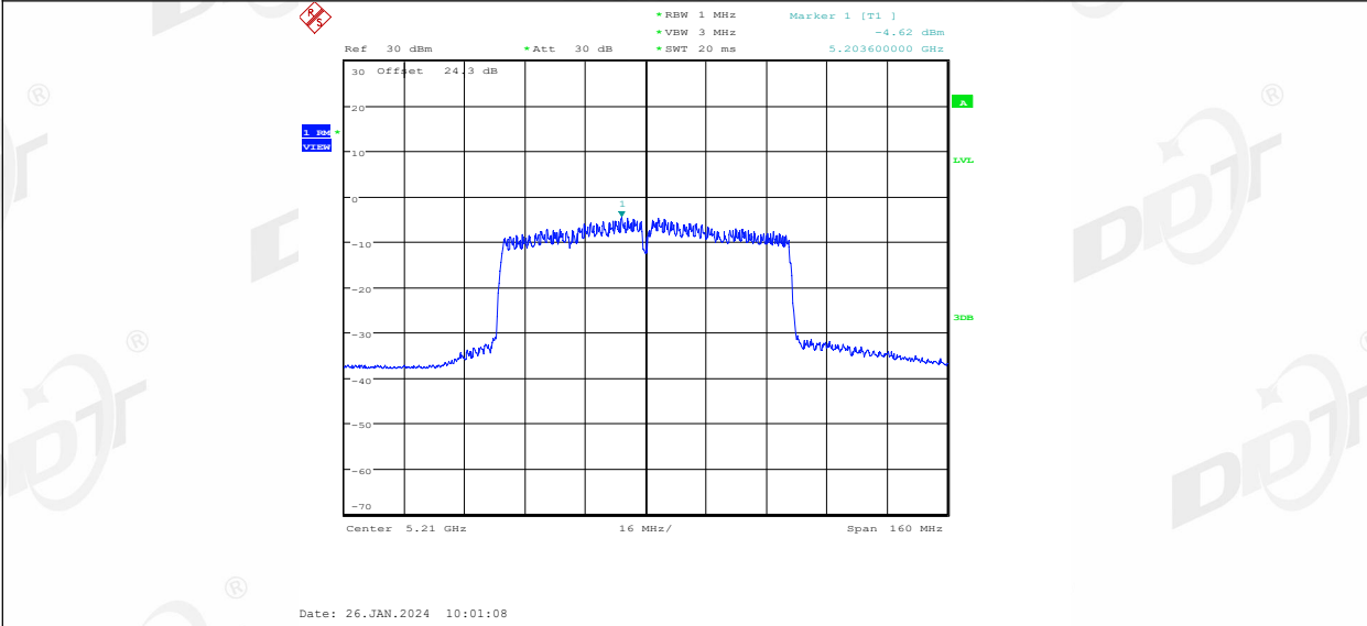
11AC80MIMO_Ant2_5210
