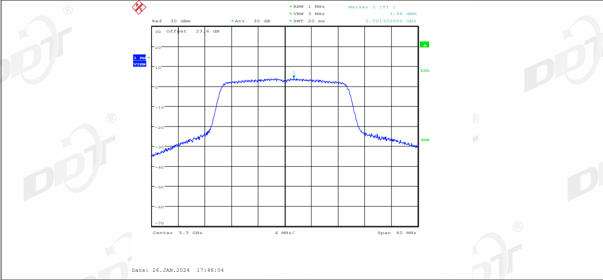
11AX20MIMO_Ant2_5500
