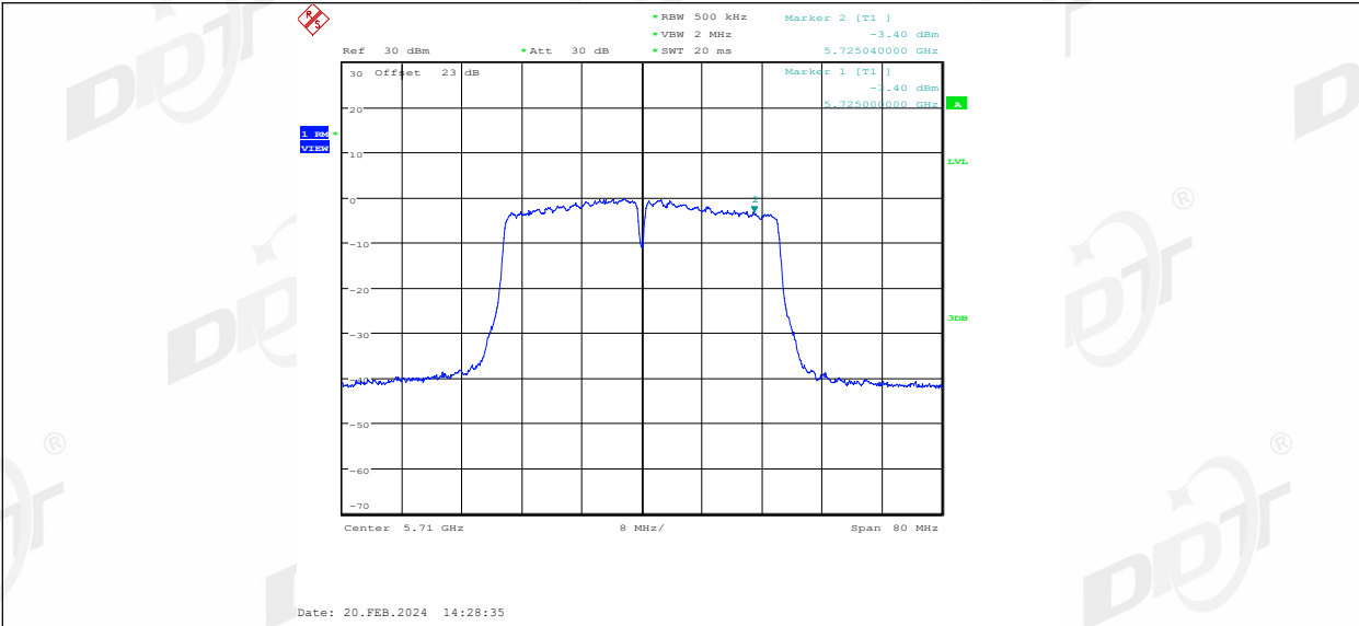
11N40MIMO_Ant2_5710_UNII-3
