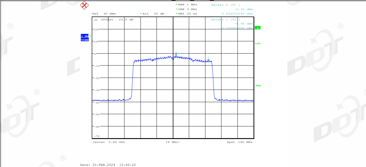
11AX80MIMO_Ant2_5690_UNII-2C
