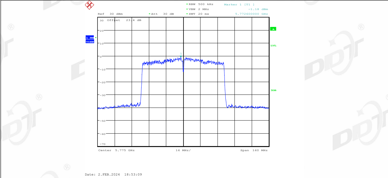
11AC80MIMO_Ant2_5775
