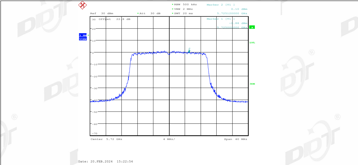
11AX20MIMO_Ant2_5720_UNII-3
