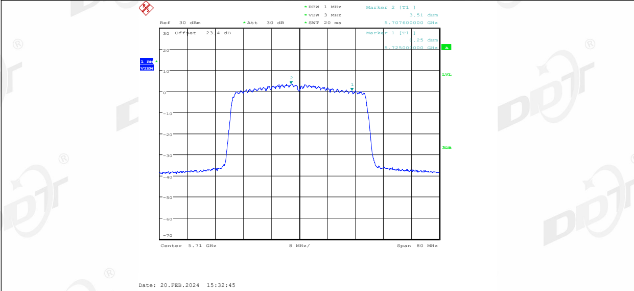
11AX40MIMO_Ant1_5710_UNII-3
