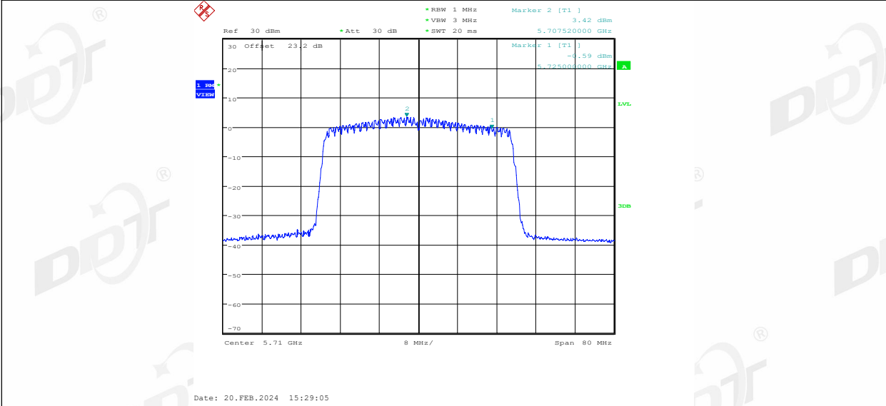
11AX40MIMO_Ant2_5710_UNII-2C
