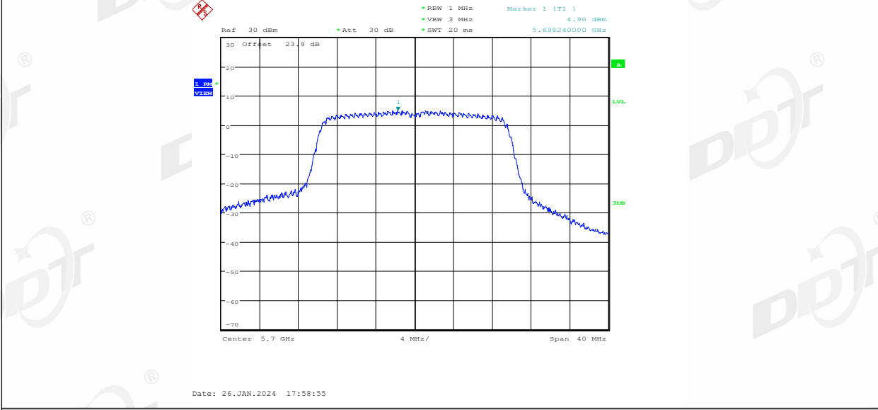
11AX20MIMO_Ant2_5700
