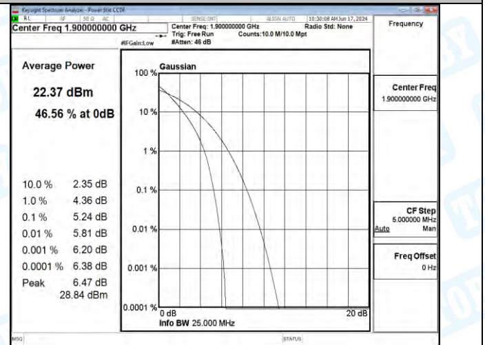
Band2-20MHz-16QAM-18700-27RB#0-PASS
